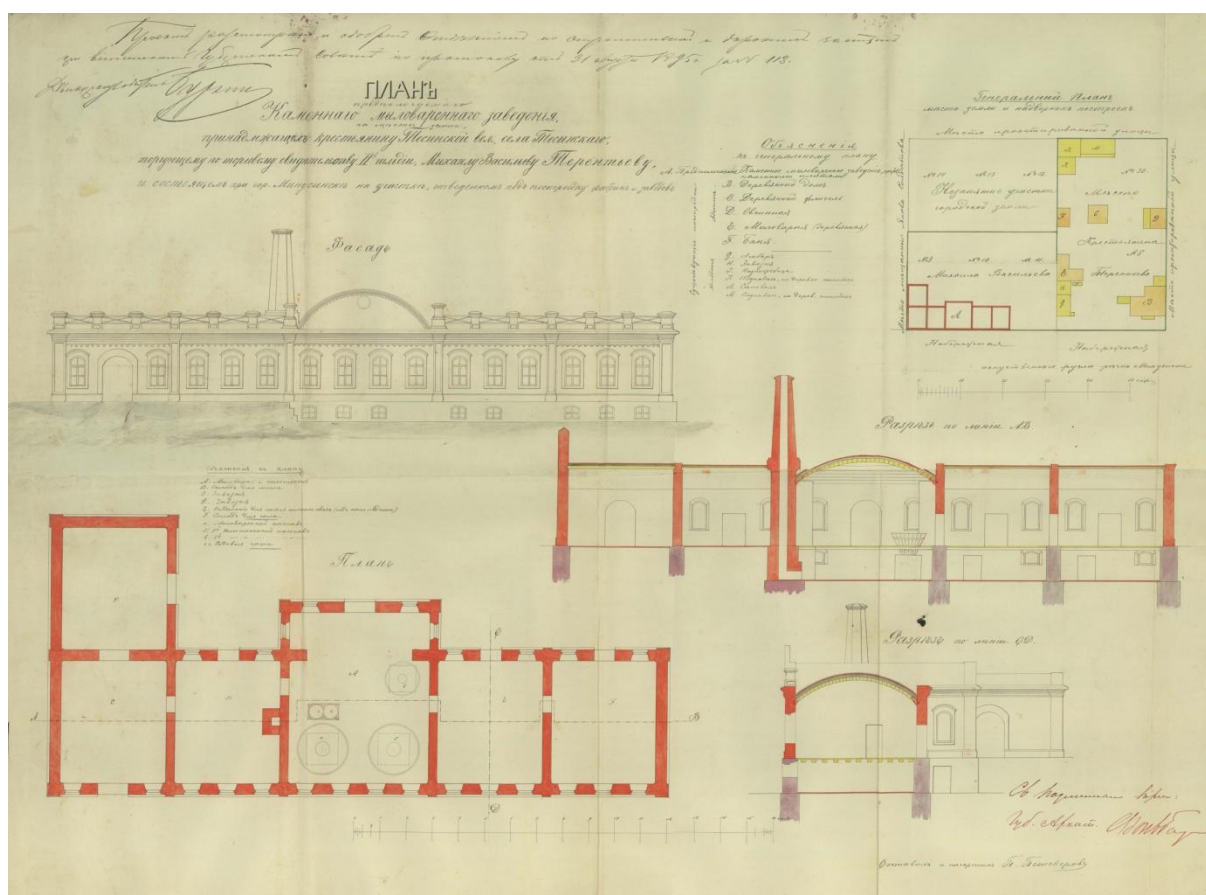
Рис. 2. План каменного мыловаренного заведения М. В. Терентьева в городе Минусинске. 1895 г. Государственный архив Красноярского края
