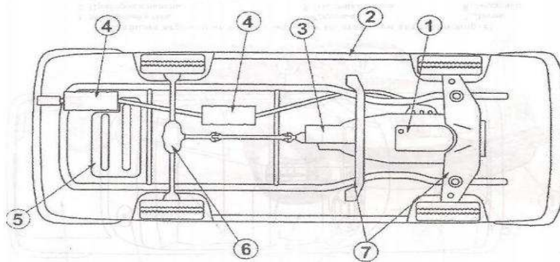
Наиболее вероятные места сокрытия на легковом автотранспорте: 1. Масляный поддон 4. Выхлопная труба 7. Все закрытые полости 2. Двери рамы 5. Бензобак 3. Механизмы 6. Распределительные механизмы
