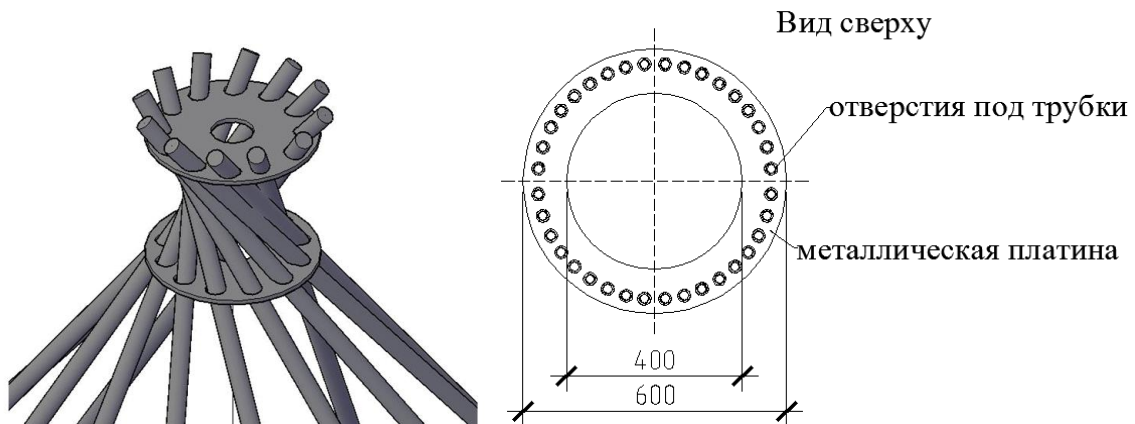
Рис.4. Верхний поворотный узел
