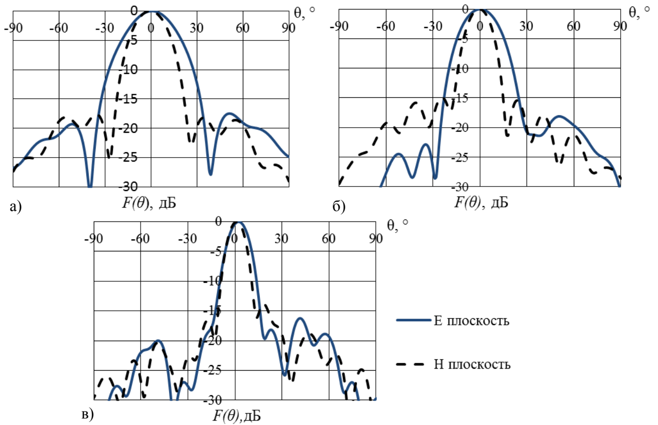
Рисунок 12 – Диаграммы направленности в E и H плоскостях на частотах а) 0,7f_0 ; б) f_0 ; в) 1,4f_0 .
