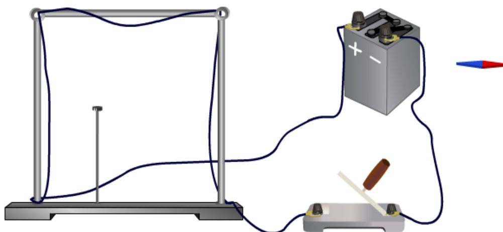
Рисунок 5. Модель «Опыт Эрстеда»
