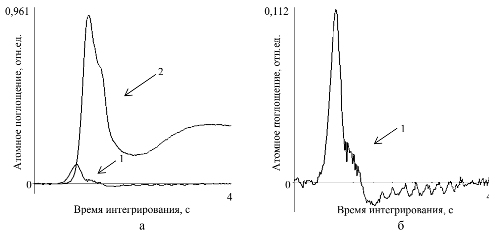
Рис. 1. Сигналы атомного (1) и фонового поглощения (2) в фосфатных буферных экстрактах для пробы почки лабораторной крысы с добавкой 11 мкг/л свинца на линии 283,3 нм (а, б)
