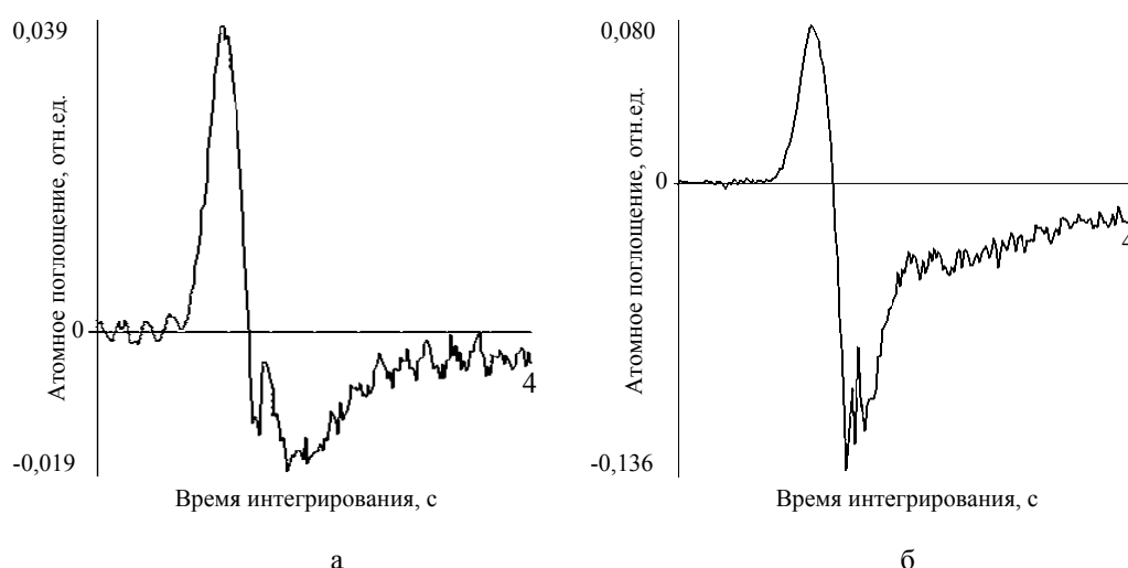
Рис. 2. Сигналы атомного поглощения для стандартного раствора свинца 5,8 мкг/л на фоне фосфатной буферной системы на линиях 283,3 (а) и 217,0 нм (б)
