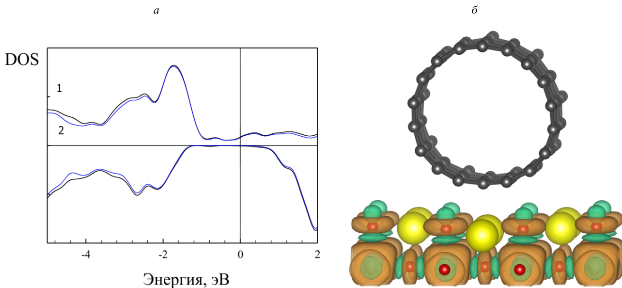
Рис. 3. Электронная структура композитов: а – плотности состояний нанокompозита CNT (9,0) / LSMO (1 – полные, 2 – парциальные плотности состояний пластины LSMO); б – пространственное распределение спиновой плотности в нанокompозите CNT (5,5) / LSMO
