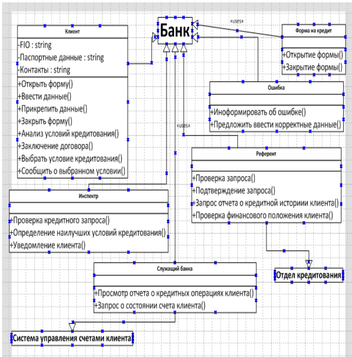
Рисунок 7 – Диаграмма классов
