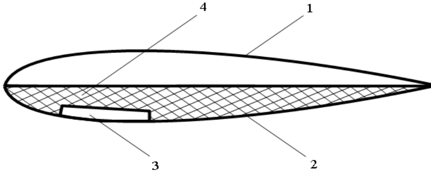
Рис. 1. Принципиальная конструкция крыла летательного аппарата противопожарной и геологоразведочной авиации, основанная на акустоэнергетическом способе увеличения подъемной силы
