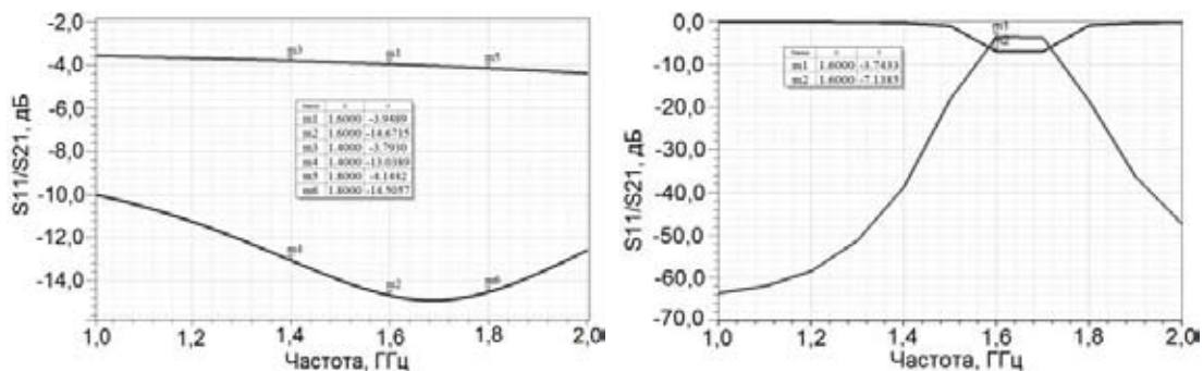
Рис. 4. S11- и S21-характеристики делителя мощности (а) и ППФ (б)
