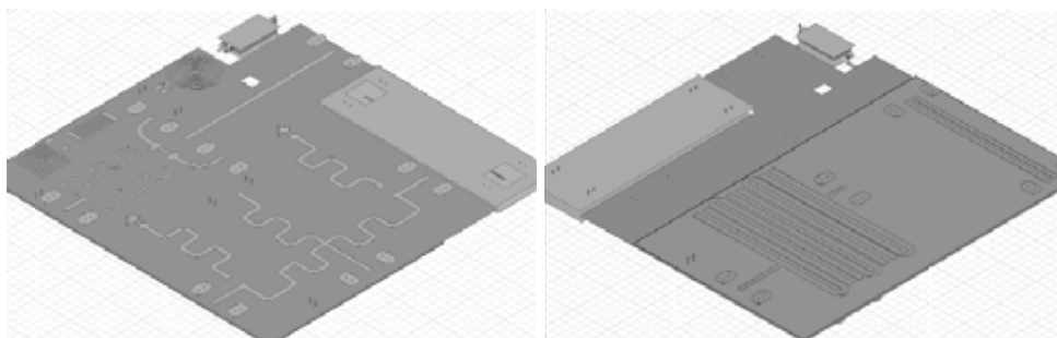
Рис. 8. Макетный образец СВЧ МИС НТК
