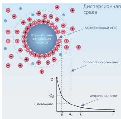
Рис.1 – Строение двойного электрического слоя (д.э.с.)
