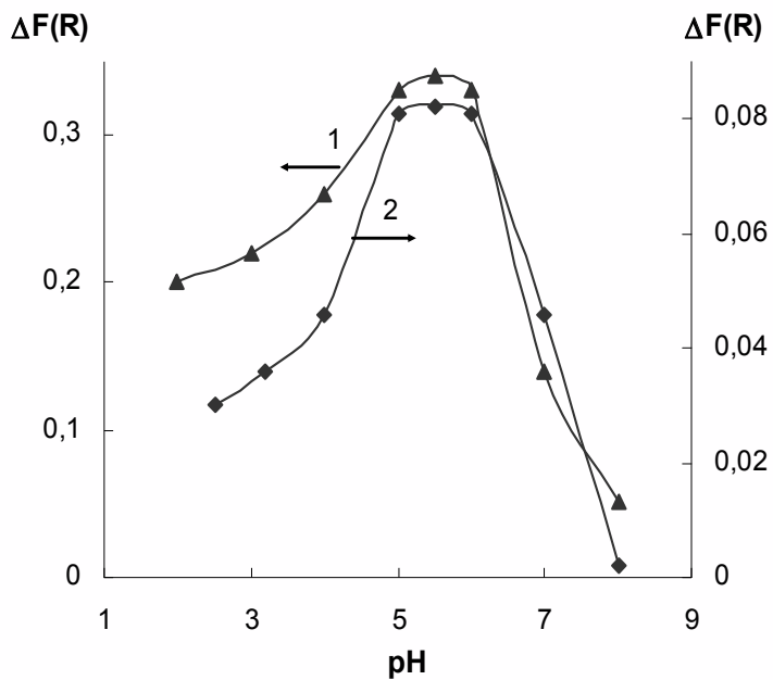
Рис. 2. Зависимости \Delta F(R) поверхностного комплекса железа(II) от pH на ZrO_2 -ПГМГ-Batophen (1) и TiO_2 -ПГМГ-Batophen (2) ( C_{Fe} = 1 мкг; 0,1 г сорбента; V = 10 мл; 0,01 М NH_2OH )
