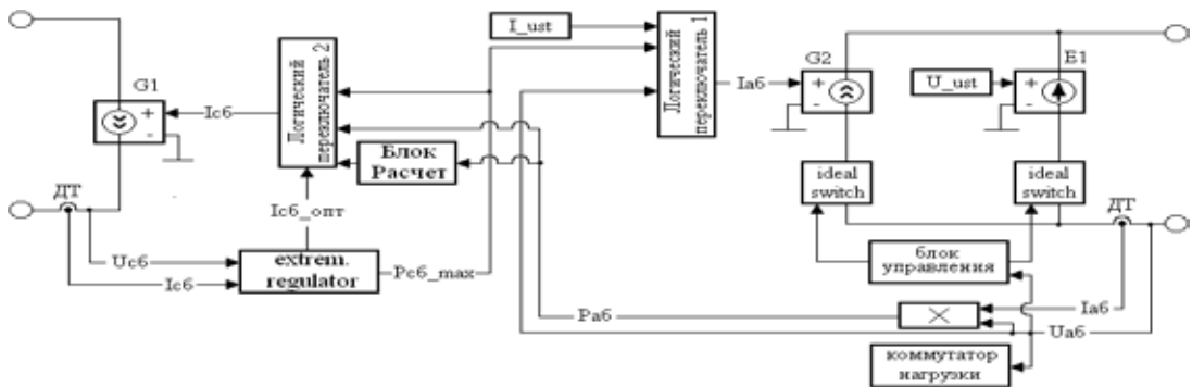
Рис. 2. Структурная схема имитационной модели контроллера солнечной батареи
