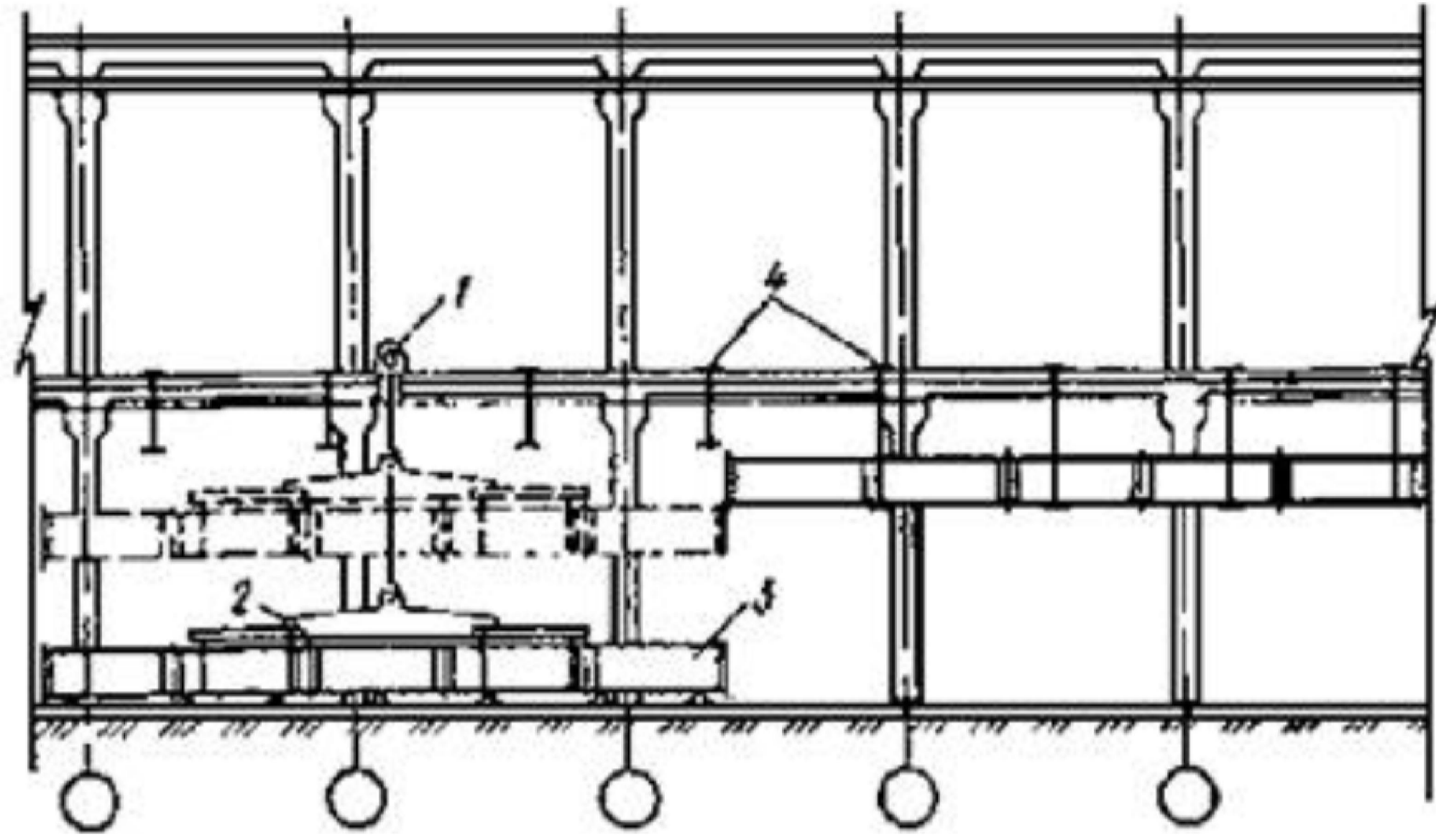
1 - лебедка; 2 - траверса; 3 - укрупненный узел воздуховода; 4 - подвески
