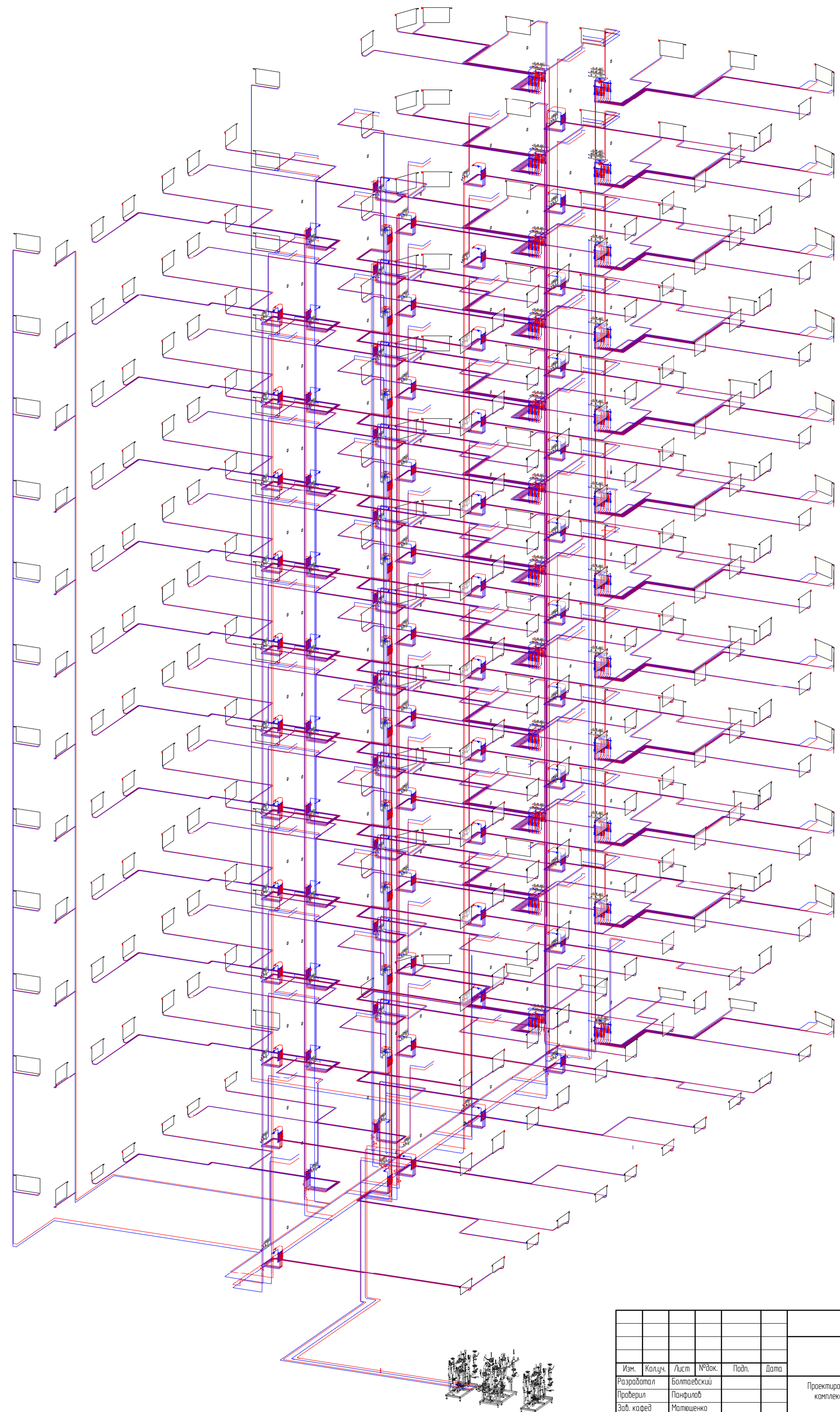
Аксонетричка схема
