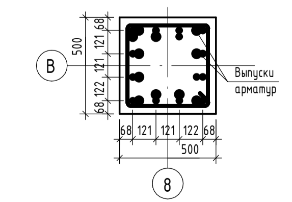
Разрез Б-Б (К-1)
