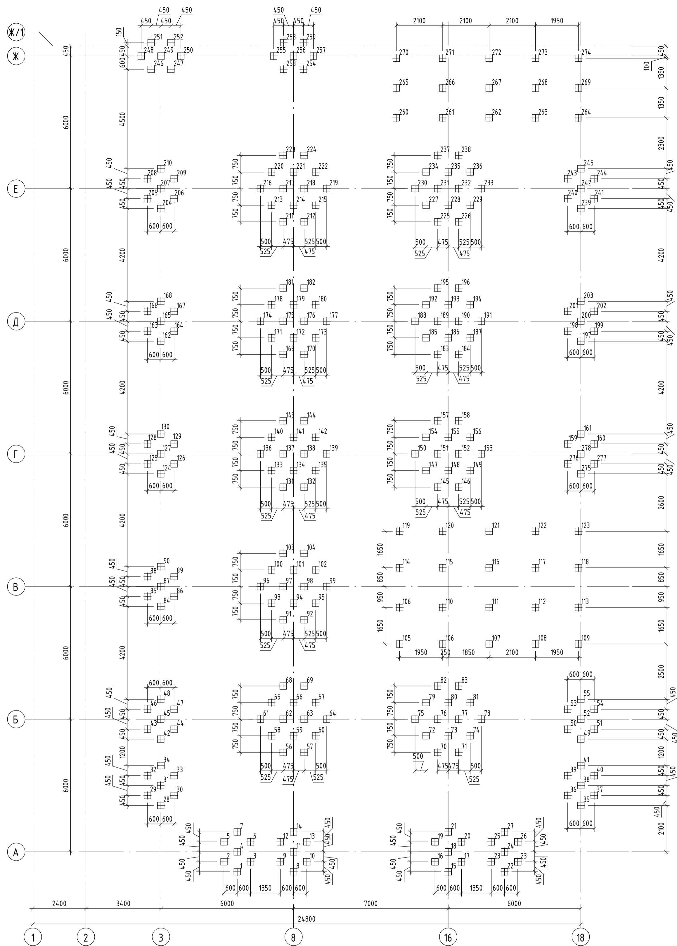
План свайного поля
