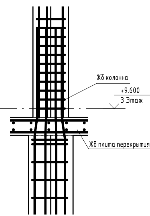
Узел примыкания жб колонны с жб плитой перекрытия
