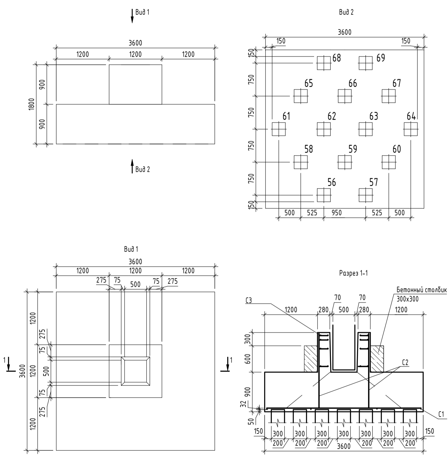
Экспликация ростверка
