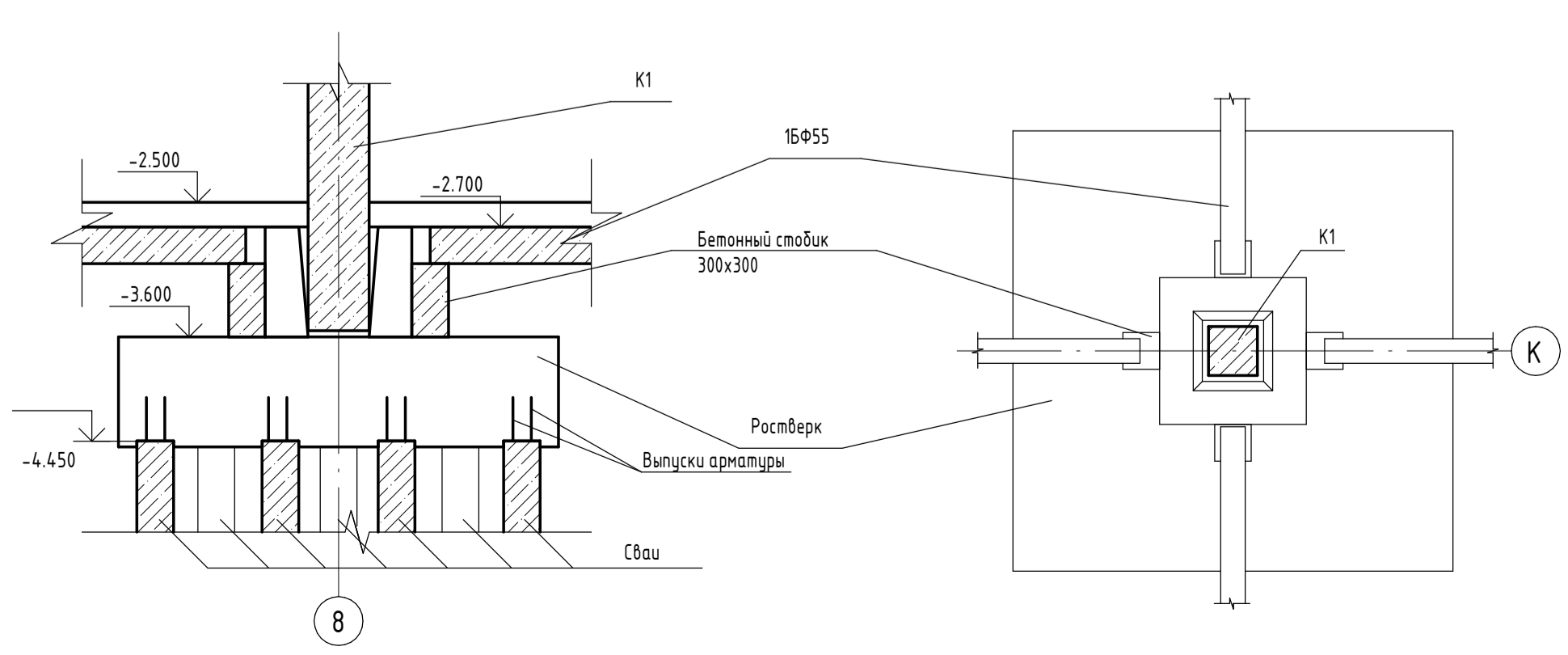
Сопряжение фундаментных балок с ростверком
