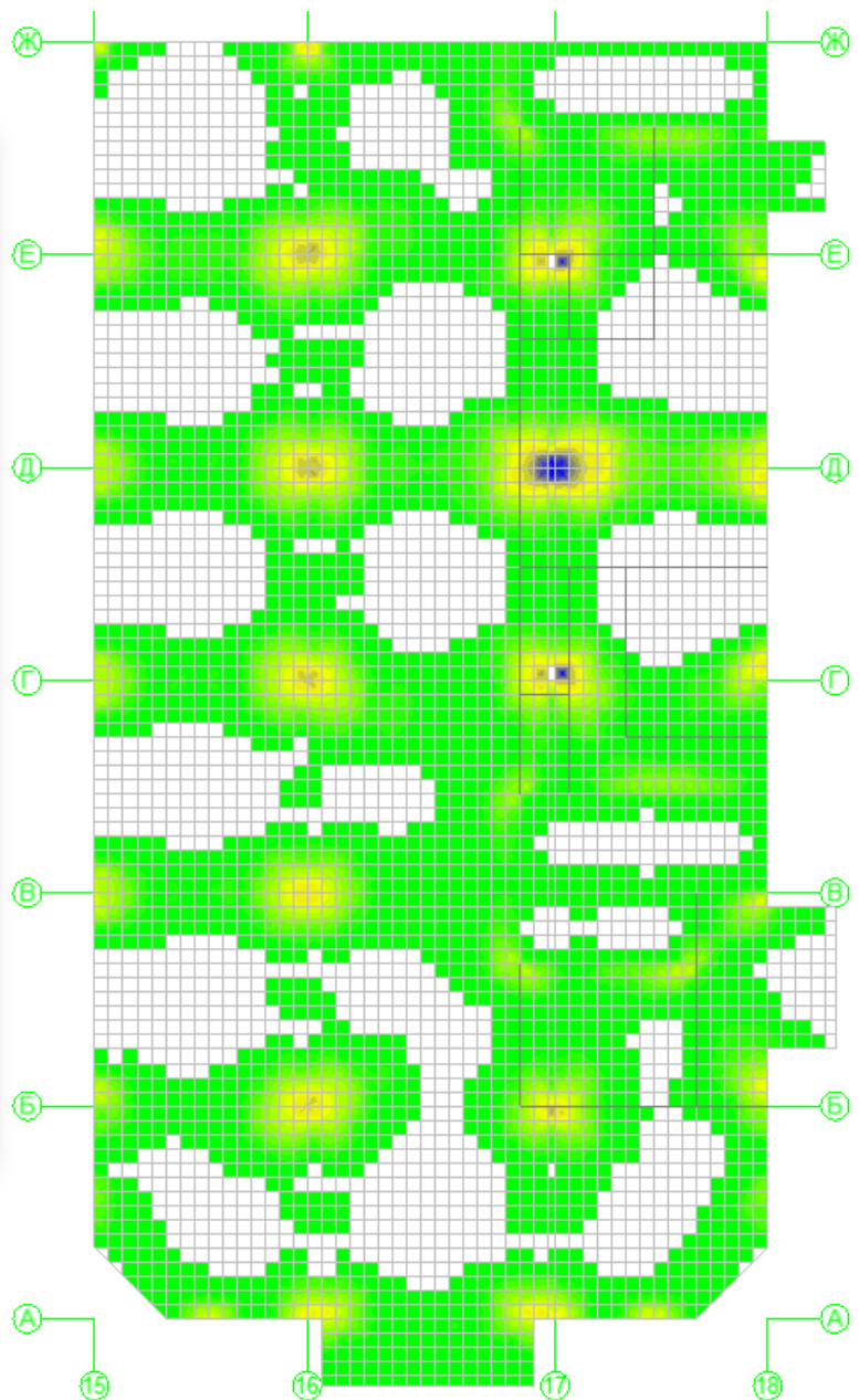
Рисунок 2.19 - Верхняя арматура вдоль цифровых осей
