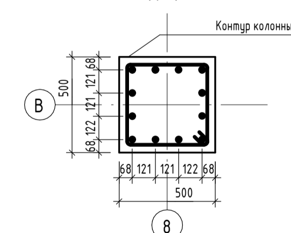
Разрез А-А К-1
