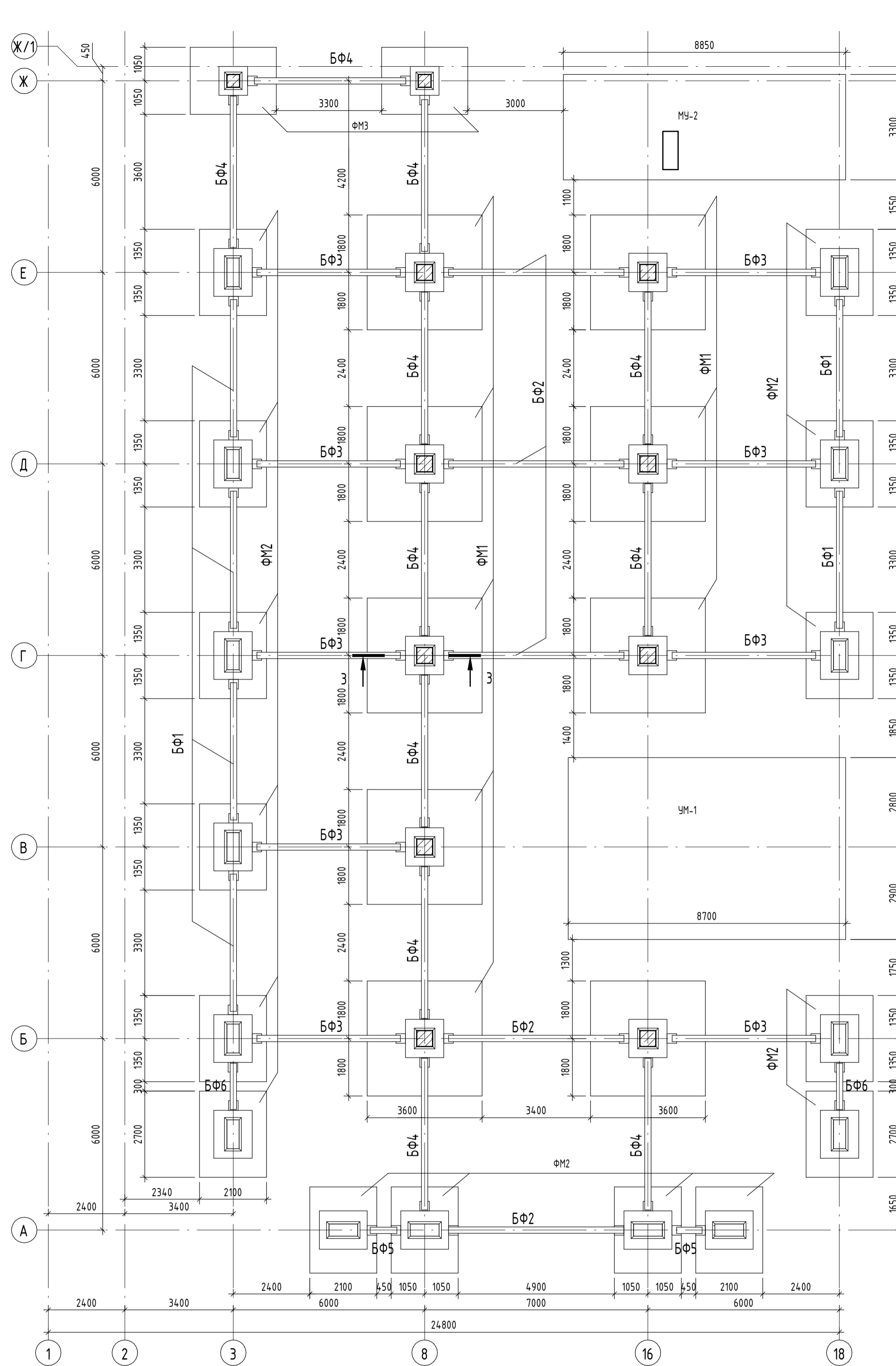
План ростверка
