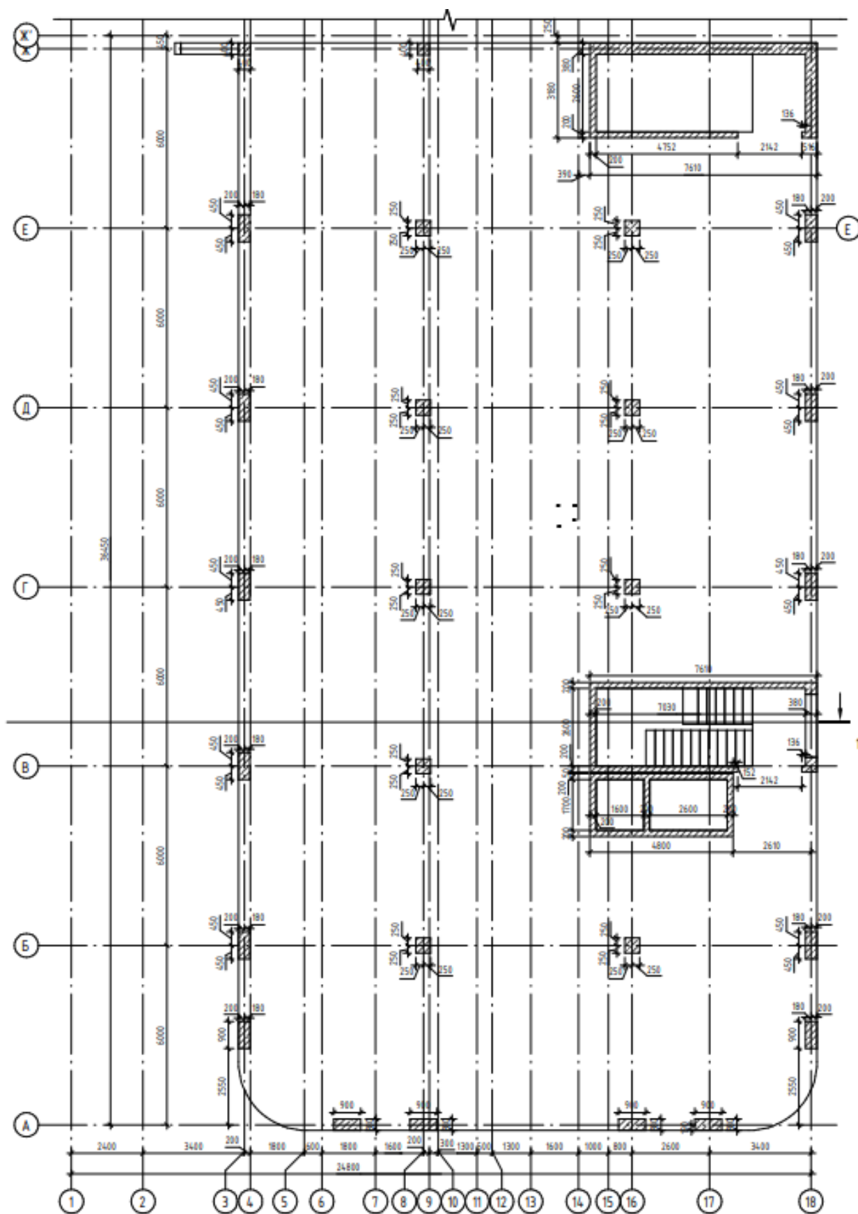
Рисунок 2.9 – Рассматриваемая плита перекрытия первого этажа
