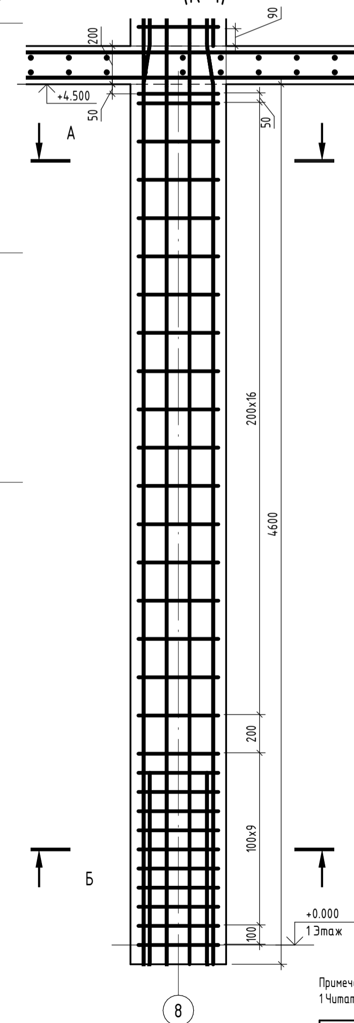
Разрез 2-2 (К-1)
