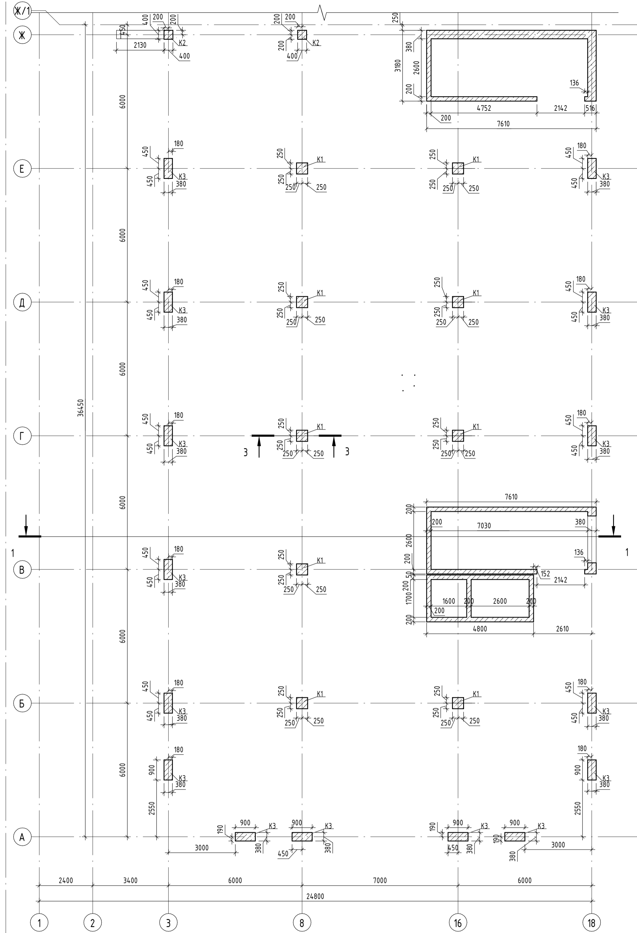
Схема расположения колонн 1 этажа
