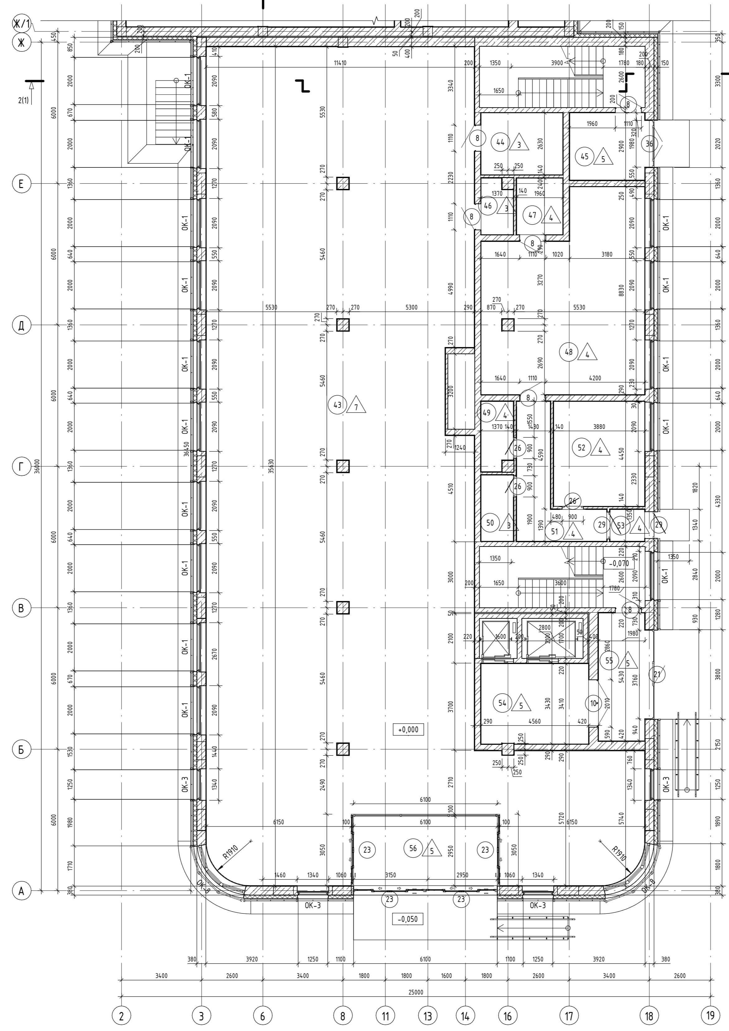
План на отм. 0,000 в осях А-Ж
