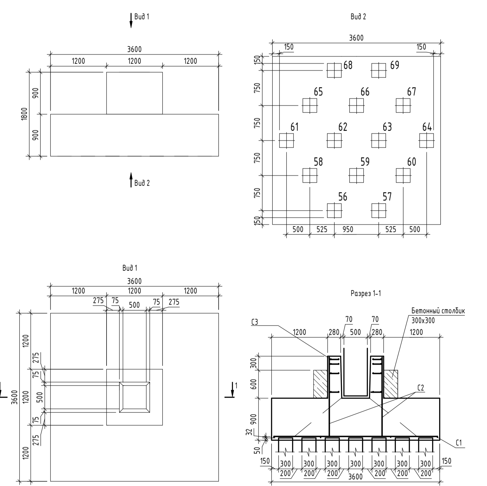
Экспликация ростверка
