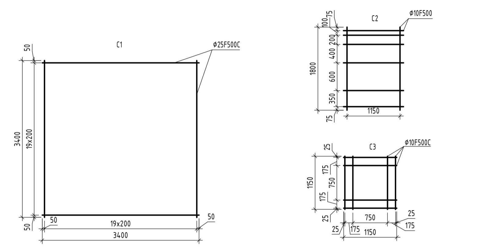
Экспликация ростверка
