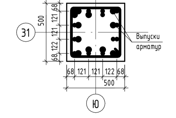
Разрез Б-Б (К-1)
