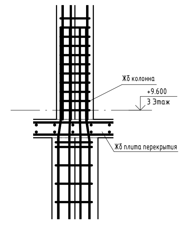
Узел примыкания жб колонны с жб плитой перекрытия
