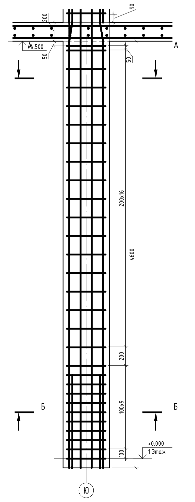
Разрез 2-2 (К-1)
