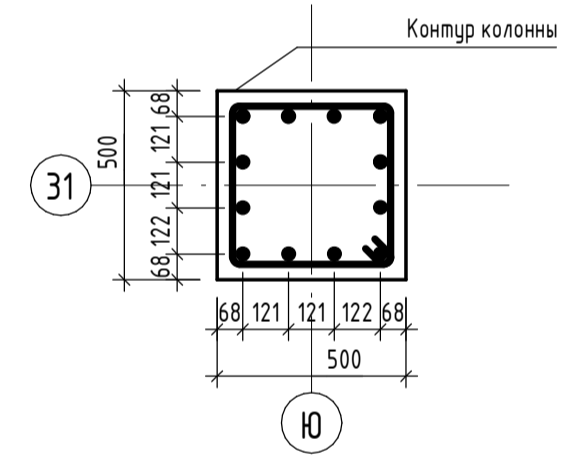
Разрез Б-Б (К-1)
