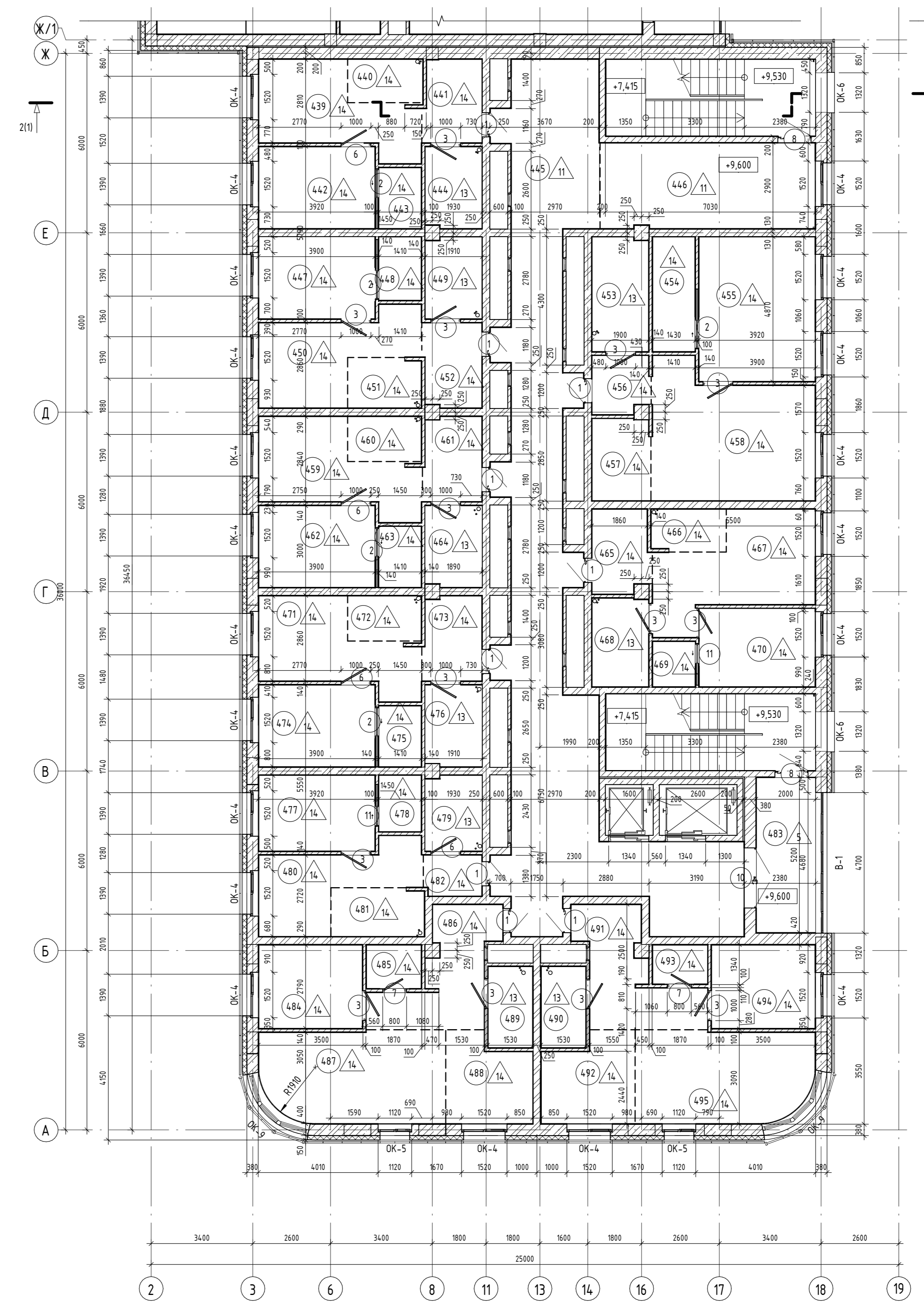
План на отм. +9,600 в осях А-Ж
