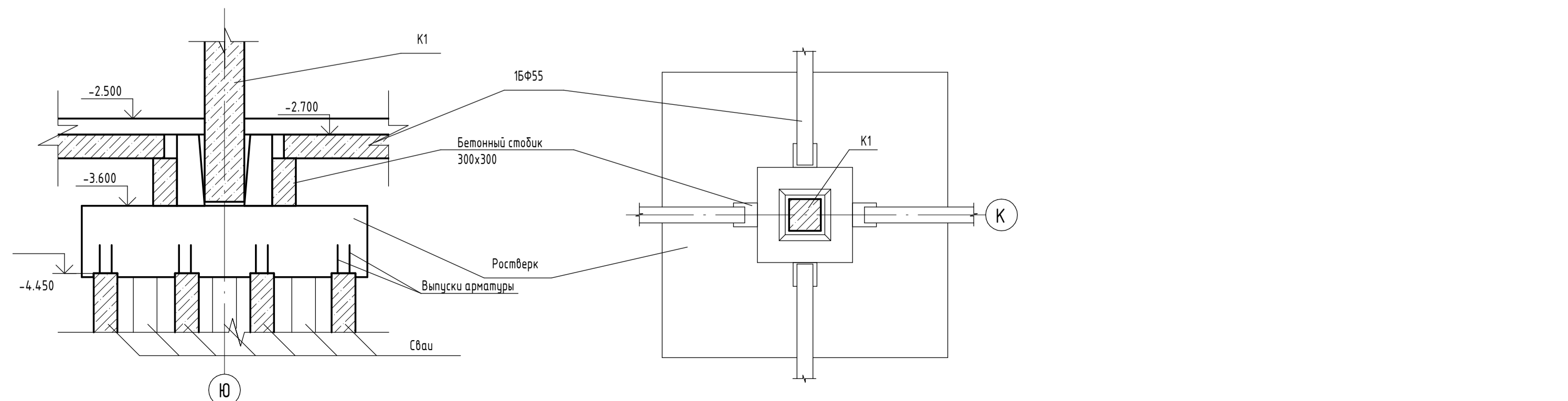
Сопряжение фундаментных балок с ростверком
