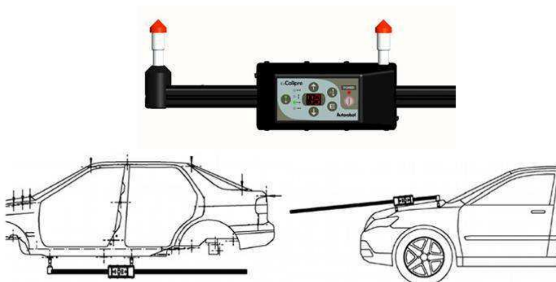
Рисунок 3.6 – Электронная измерительная линейка AutorobotEzCalipre и примеры ее применения
