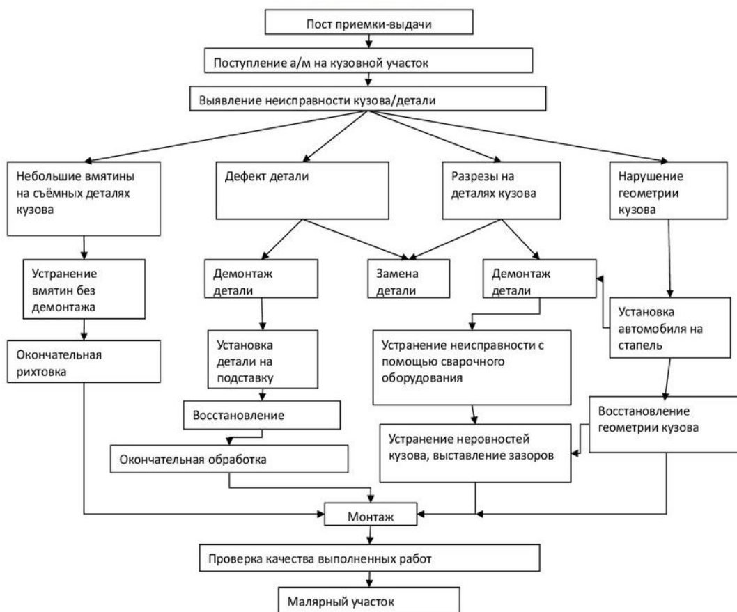
Рисунок 2.1 – Схема технологического процесса ремонта кузова автомобиля
