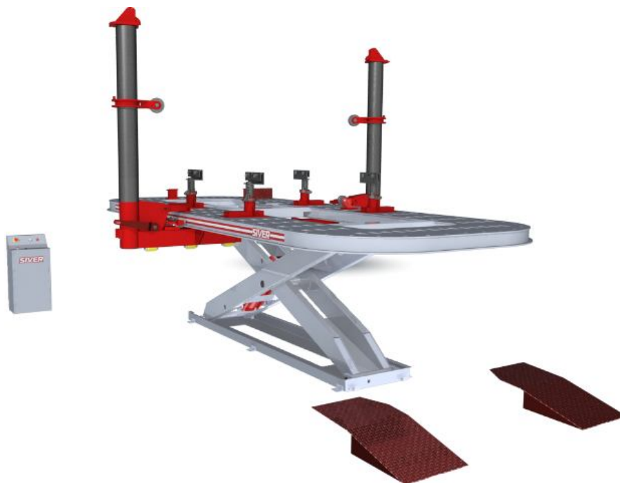
Рисунок 3.2 – Стапель SIVEREL-210
