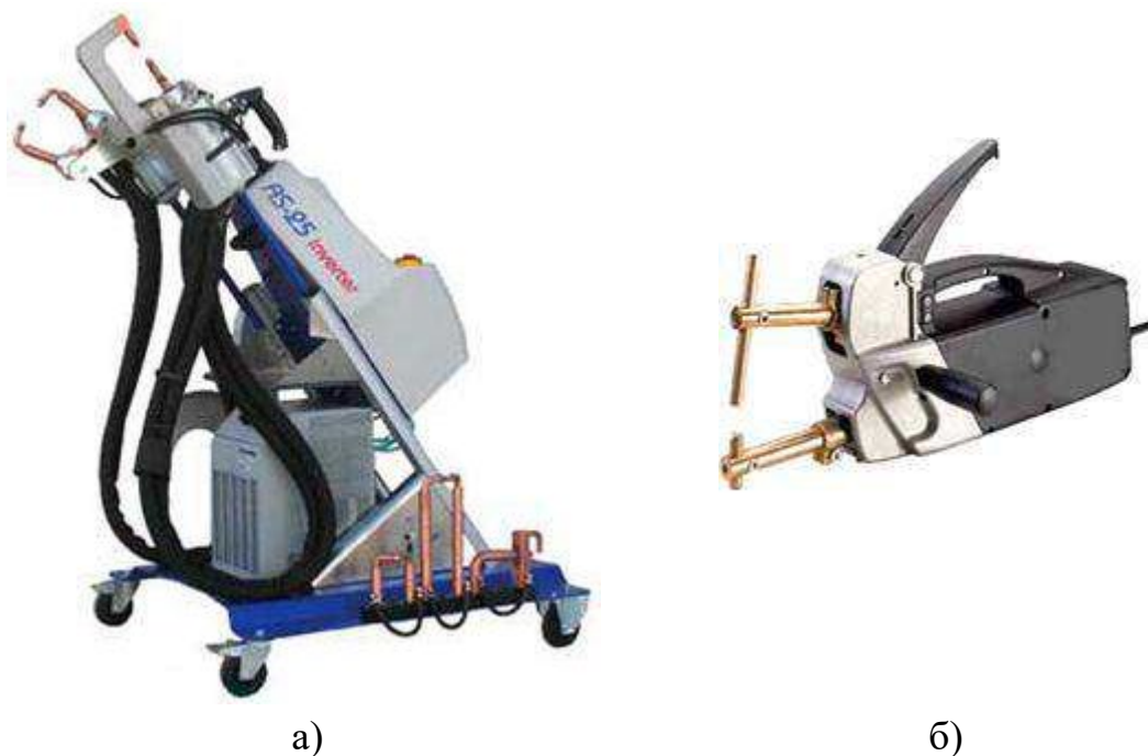
а) – мобильная многофункциональная сварочная станция CarBench AS-25-CX б) – двухэлектродный сварочный пистолет
