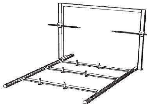
Рисунок 3.4 – Общий вид механической измерительной системы Autorobot
