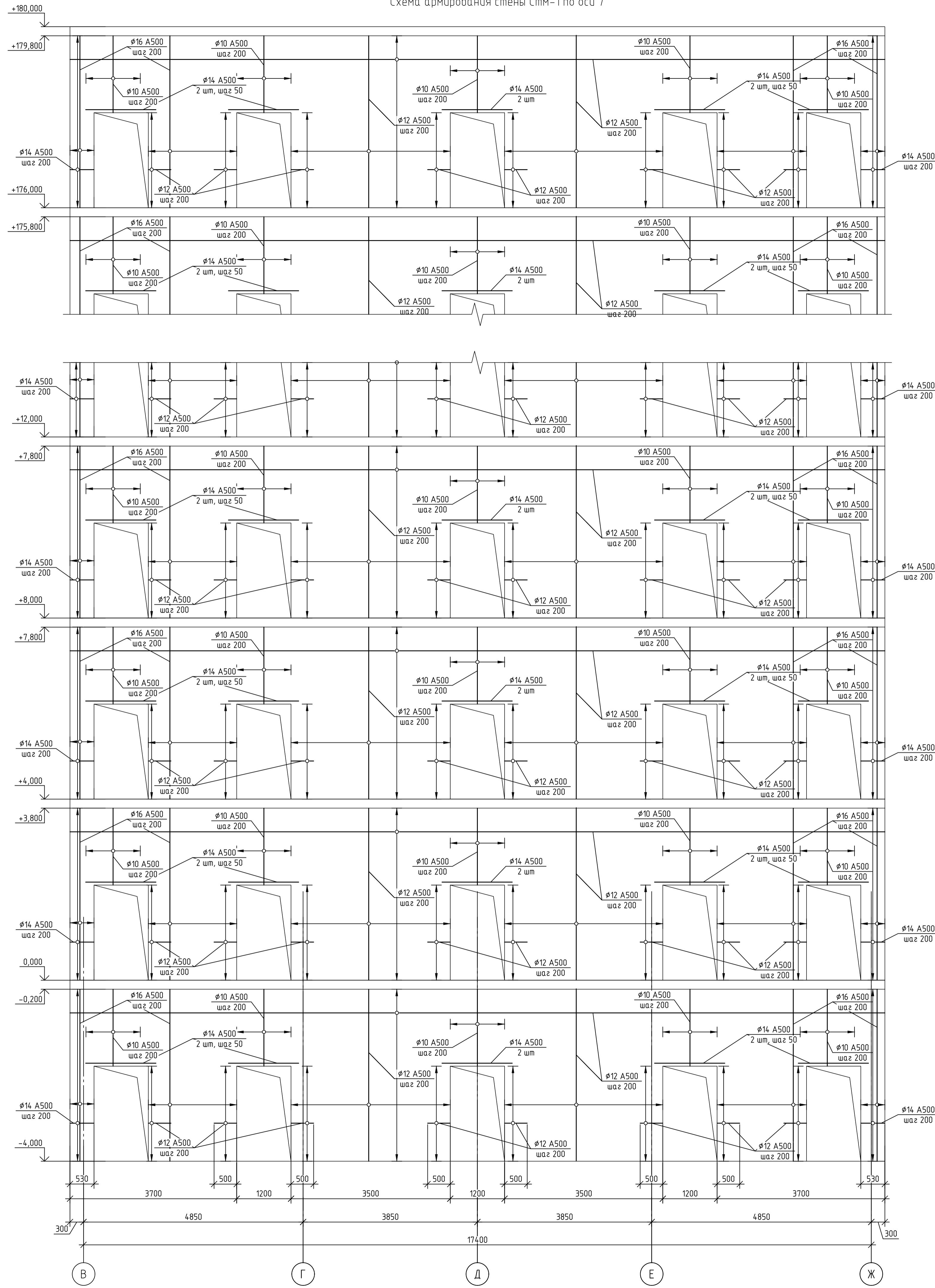
Схема армирования стены Стм-1 по оси 7
