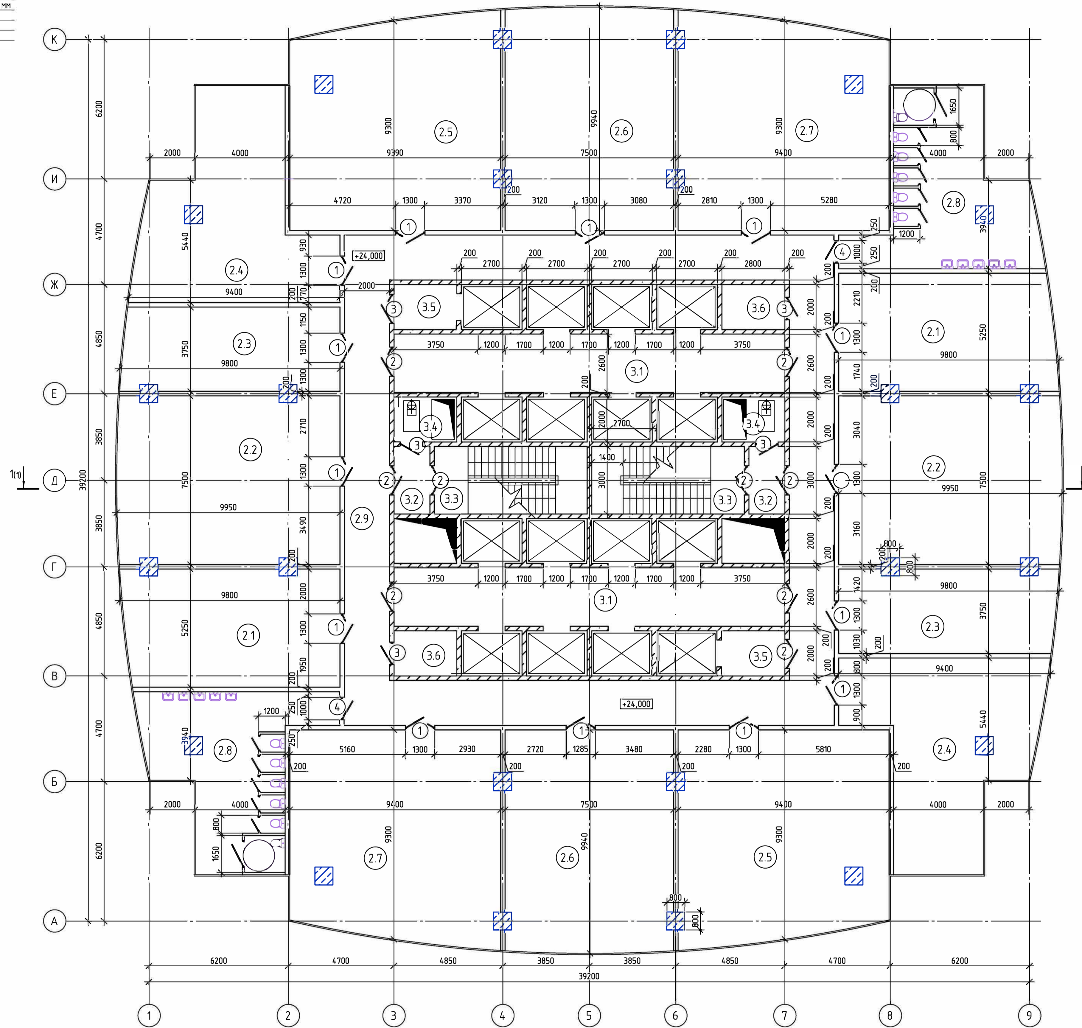
План этажа на отметке +24.000
