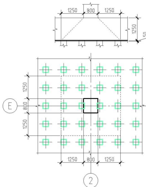
Рисунок 4.4 - Схема работы ростверка на продавливание колонной
