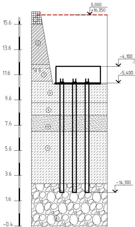
Рисунок 4.6 – Буронабивные сваи
