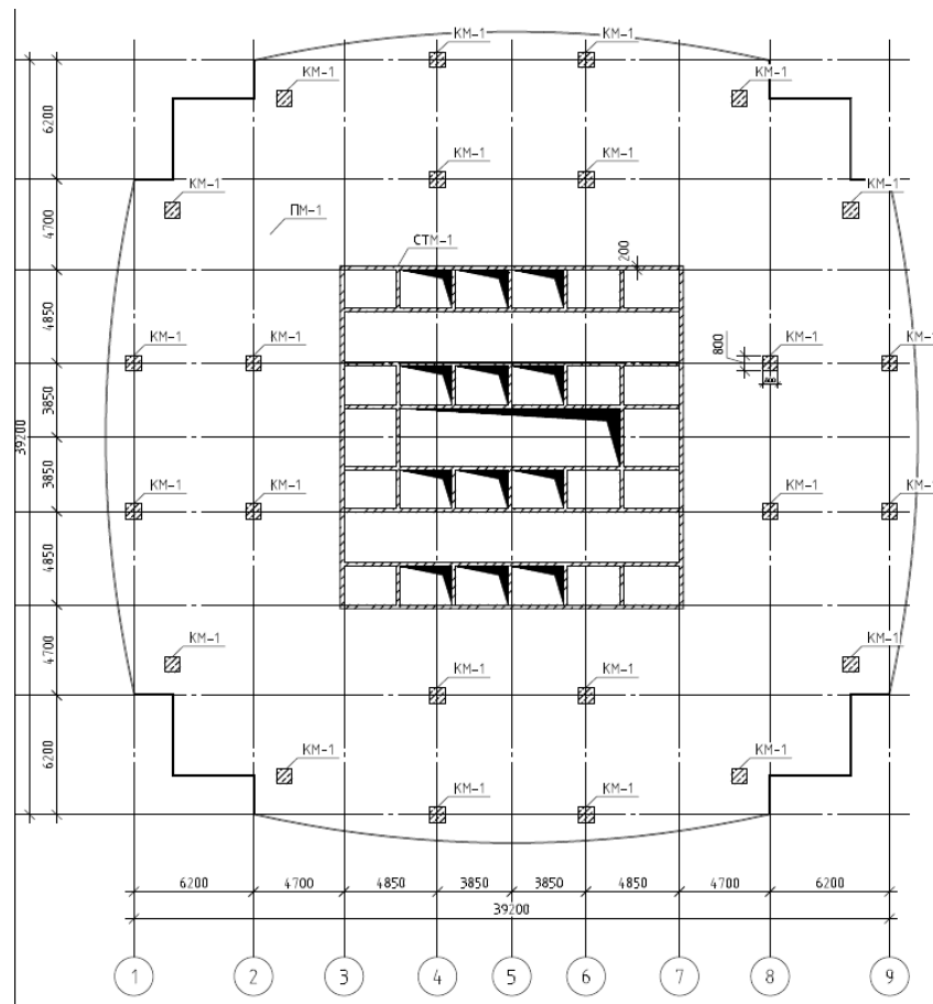
Рисунок 3.1 – Схема расположения несущих элементов
