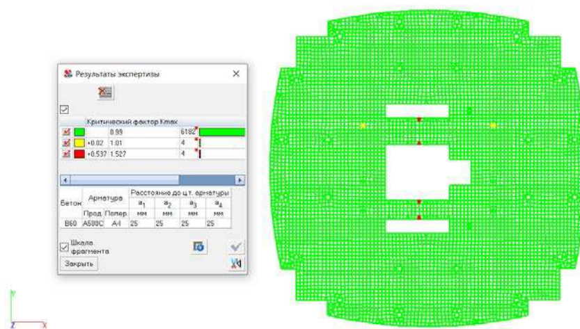
Рисунок 3.27 – Результаты экспертизы нижнего армирования плиты перекрытия
