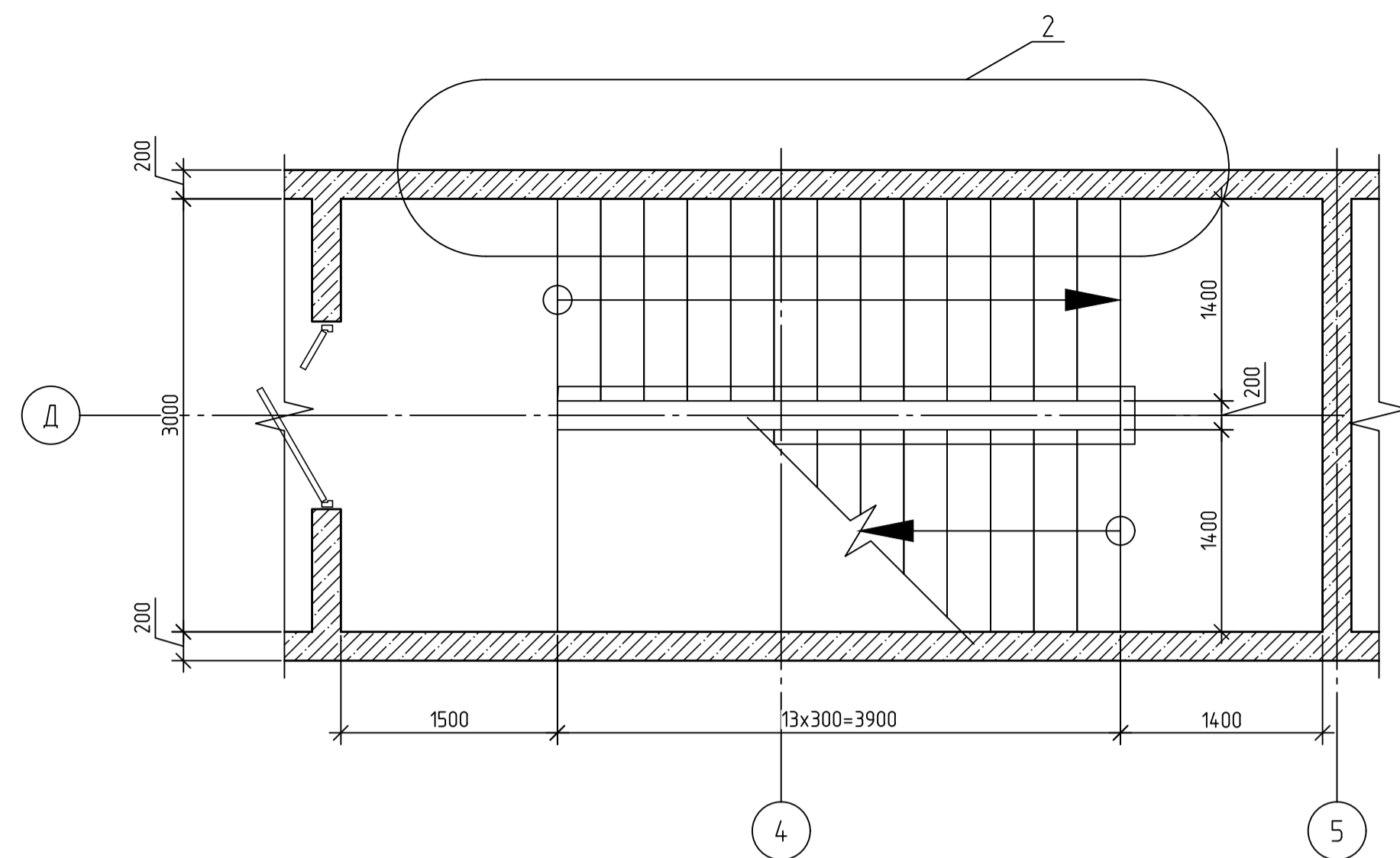
Схема расположения закладных деталей для крепления ограждения
