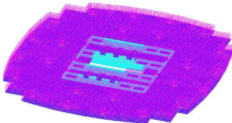
Рисунок 3.5 – Временная нагрузка на перекрытия
