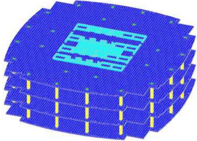
Рисунок 3.2 – Сгенерированная схема в ПК SCAD с указанием типов жесткости
