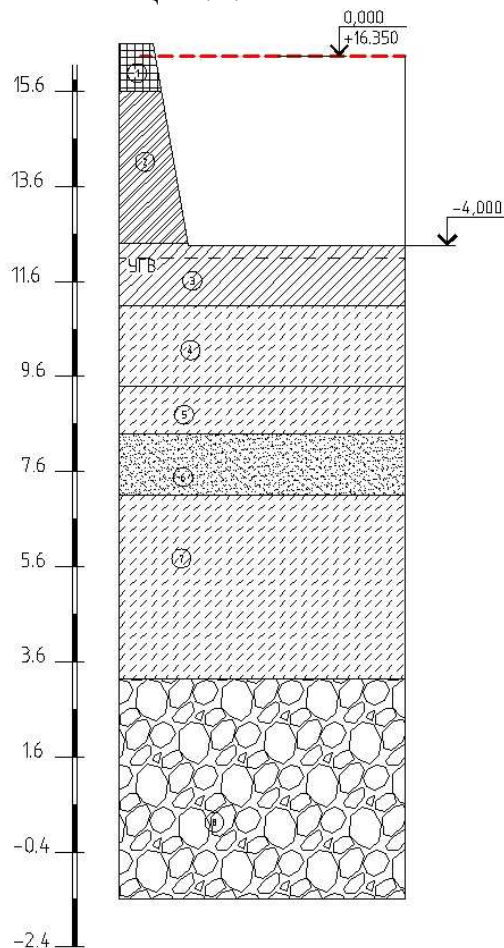
Рисунок 4.1 - Инженерно – геологическая колонка
