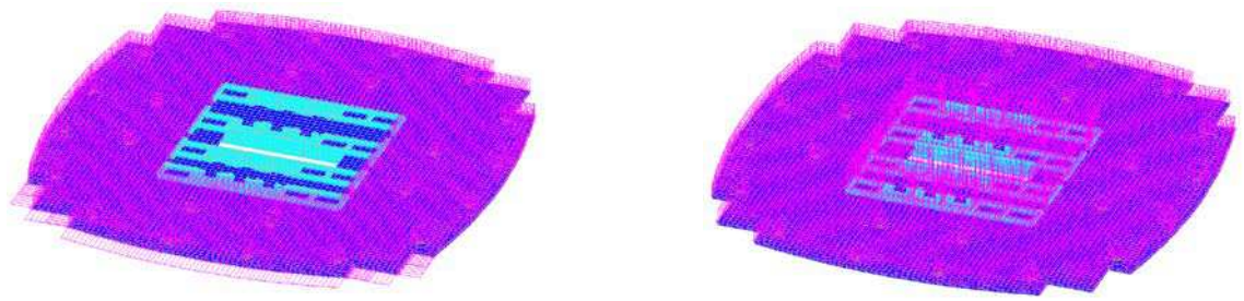
Рисунок 3.3 – Нагрузка от перегородок; рисунок 3.4 – Нагрузка от собственного веса
