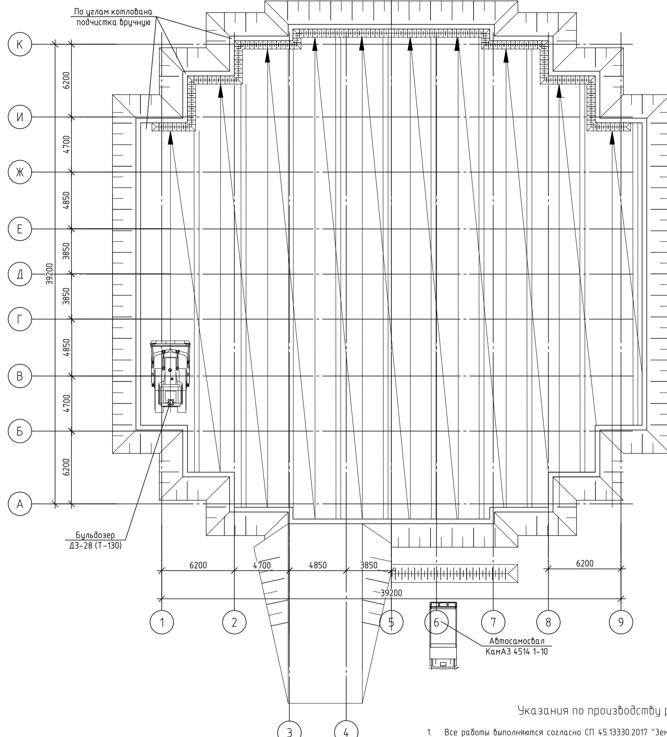
Подсыпка дна котлована
