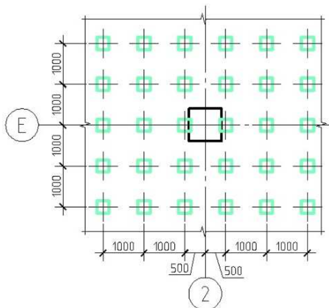
Рисунок 4.3 – Схема расположения свай под фрагмент плитного фундамента
