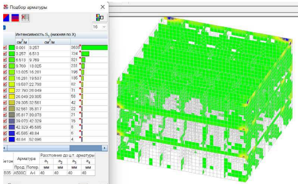
Рисунок 3.29 – Изополя армирования ядра жесткости
