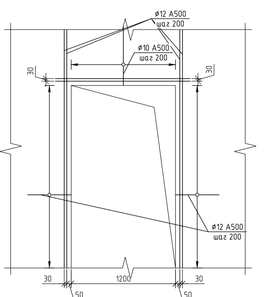
Деталь оформления проема
