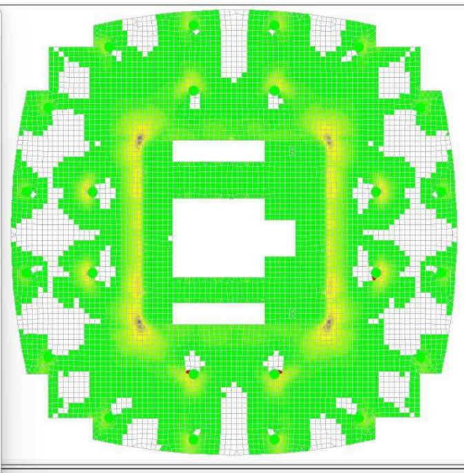
Рисунок 3.24 – Изополя армирования плиты интенсивность S_2 (верхняя по X)
