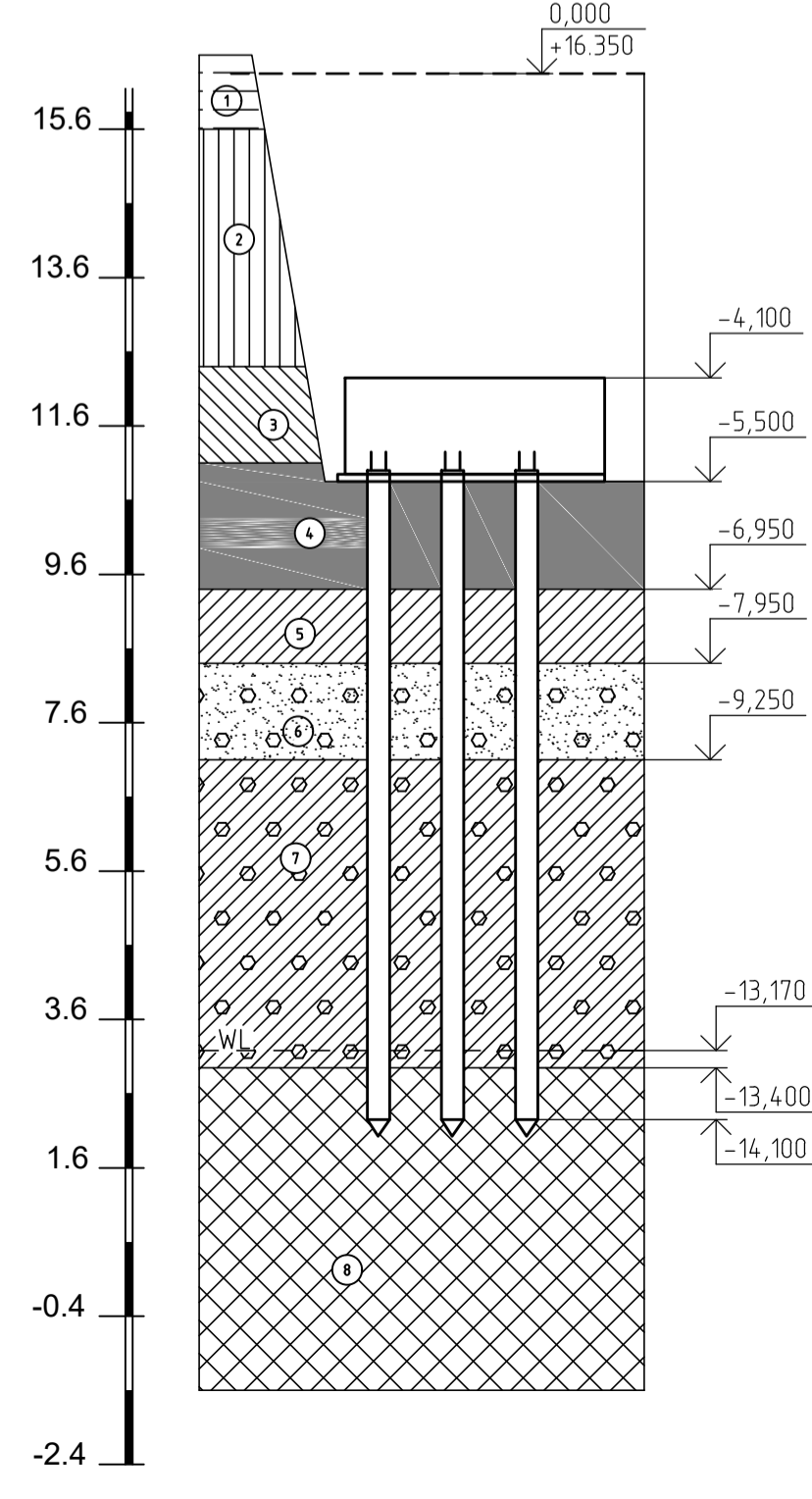
Инженерно-геологический разрез
