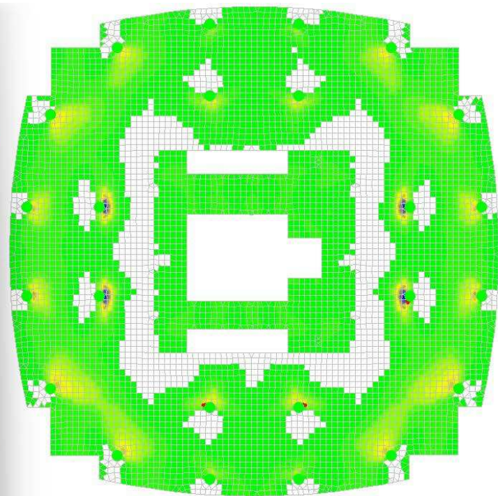
Рисунок 3.23 – Изополя армирования плиты интенсивность S_1 (нижня по X)
