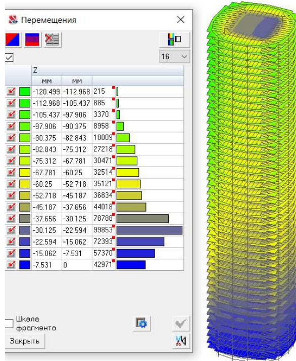
Рисунок 3.10 – Вертикальные перемещения по оси Z
