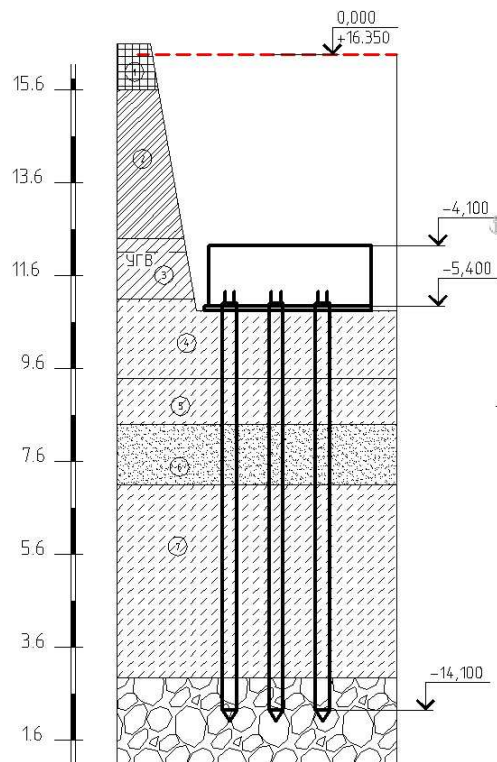
Рисунок 4.2- Забивная свая
