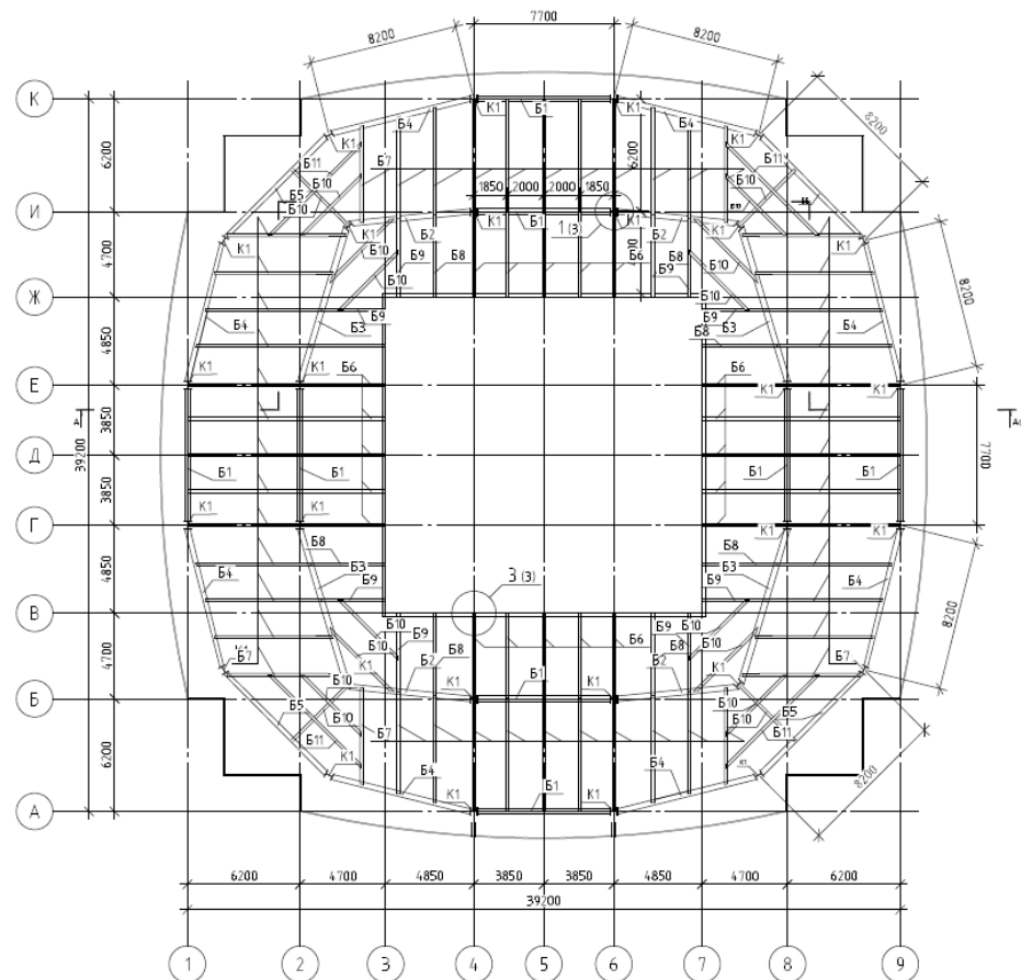
Рисунок 1.2 – План расположения несущих элементов металлического каркаса здания
