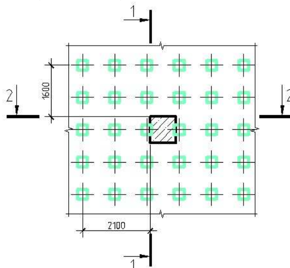
Рисунок 4.5 - Схема к расчету плиты на изгиб
