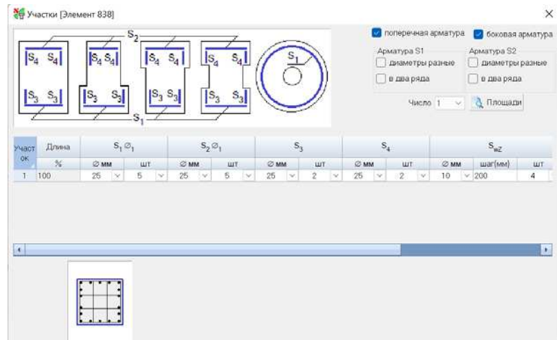
Рисунок 3.18 – Армирование колонн КМ-3 (400x400 мм)
