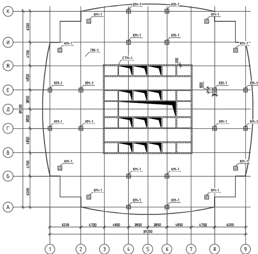
Рисунок 1.1 – План расположения несущих элементов железобетонного каркаса здания
