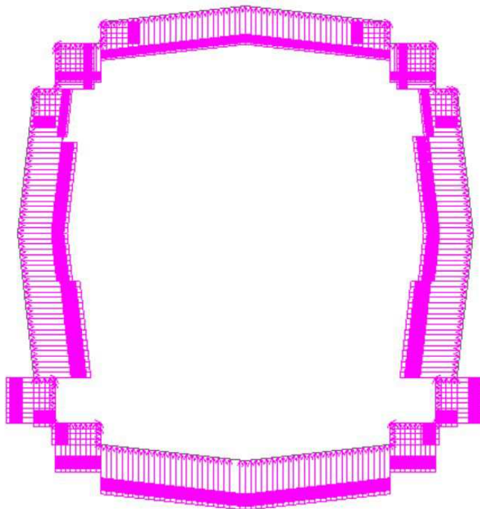
Рисунок 3.6 - Нагрузка от статической составляющей ветровой нагрузки (вдоль оси Y)
