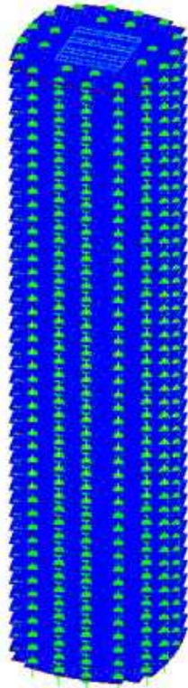
Рисунок 3.2 – Сгенерированная схема в ПК SCAD с указанием типов жесткости
