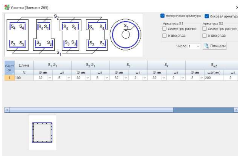
Рисунок 3.16 – Армирование колонн КМ-1 (800x800 мм)
