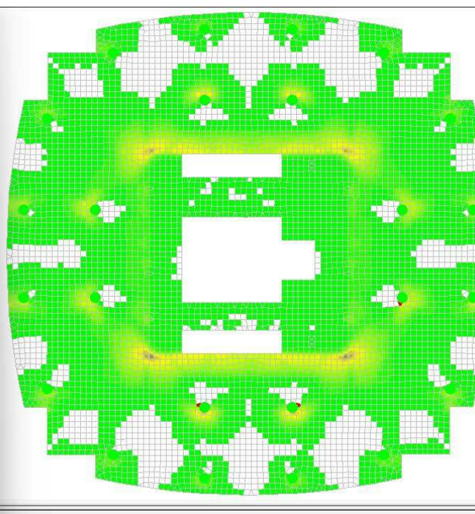
Рисунок 3.25 – Изополя армирования плиты интенсивность S_3 (верхняя по Y)
