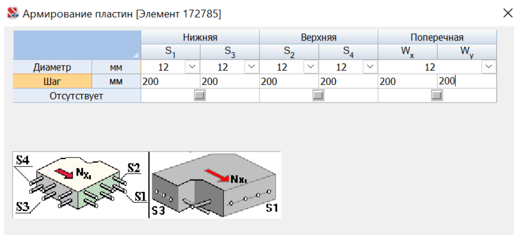
Рисунок 3.30 – Основное армирование ядра жесткости
