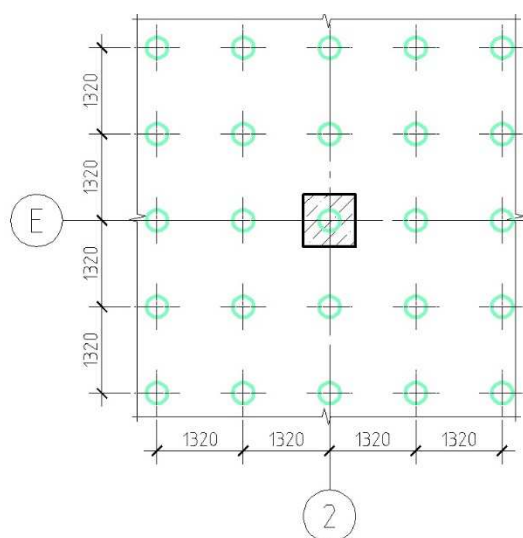
Рисунок 4.7 – Схема расположения свай под фрагмент плитного фундамента
