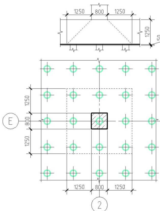
Рисунок 4.8 - Схема работы ростверка на продавливание колонной
