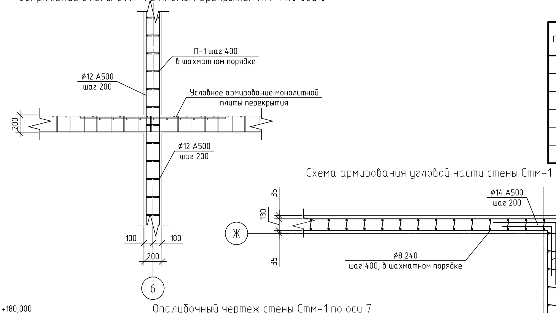
Сопряжение стены Стм-1 и плиты перекрытия ПМ-1 по оси 6
