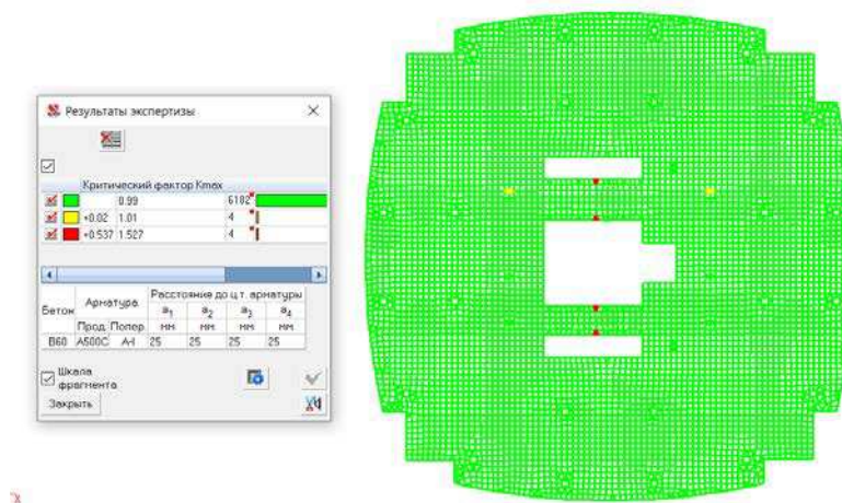
Рисунок 3.28 – Результаты экспертизы верхнего армирования плиты перекрытия
