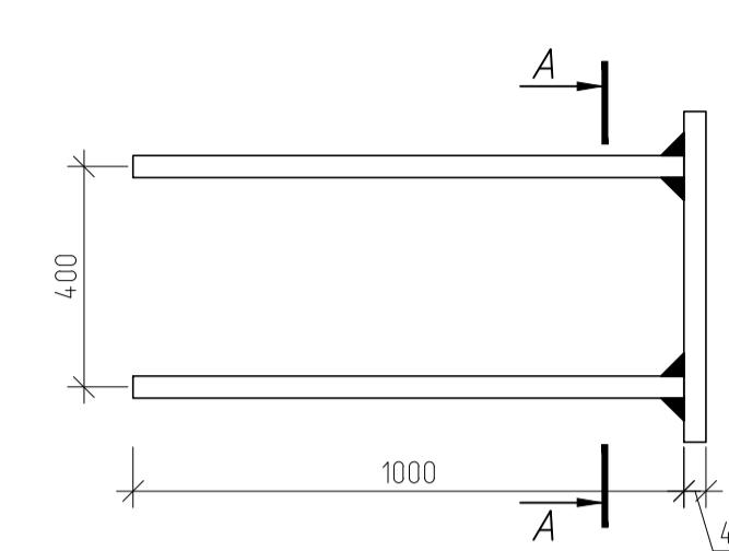
Закладная деталь Зб-1
