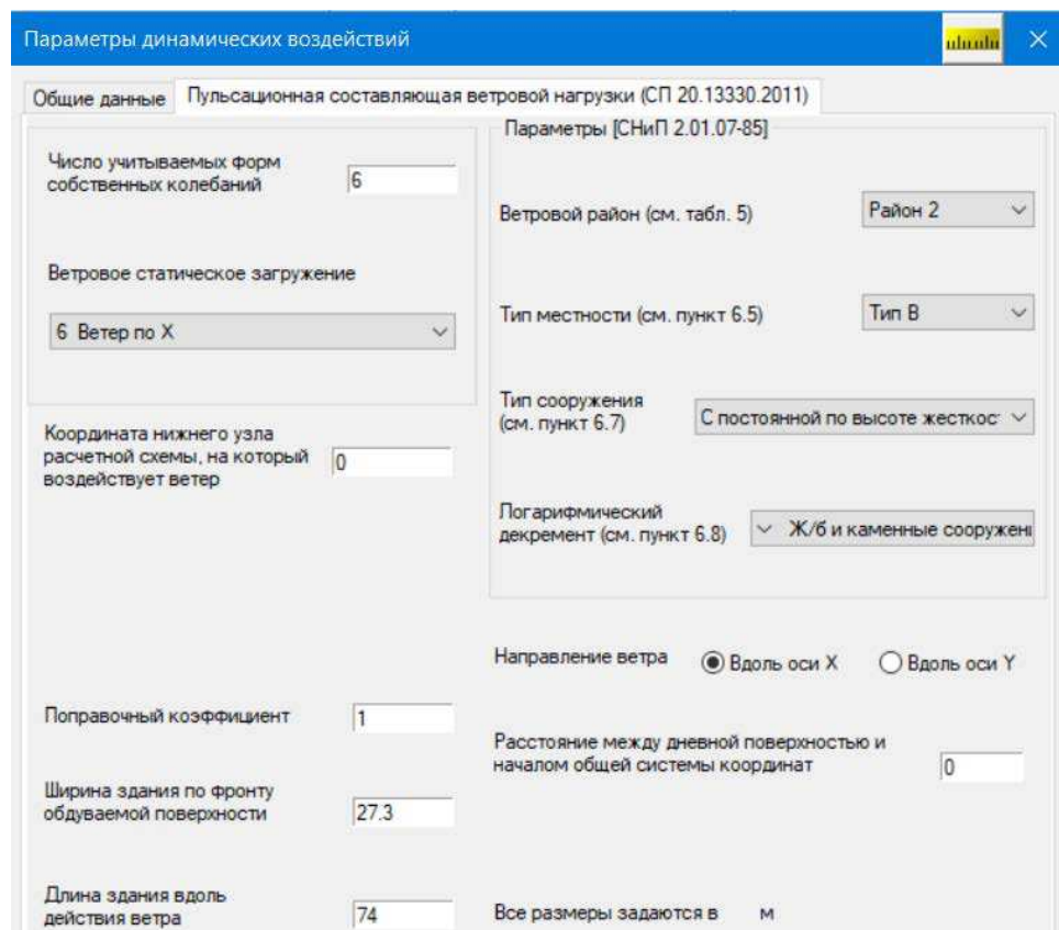
Рисунок 3.8 – Параметры динамического воздействия
