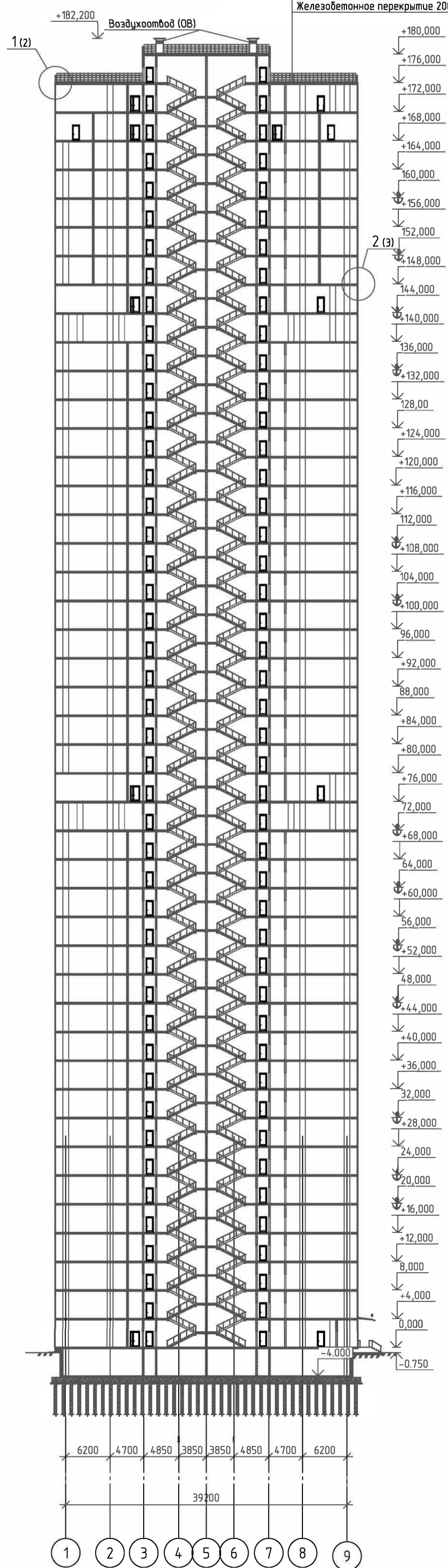
Разрез 1-1
