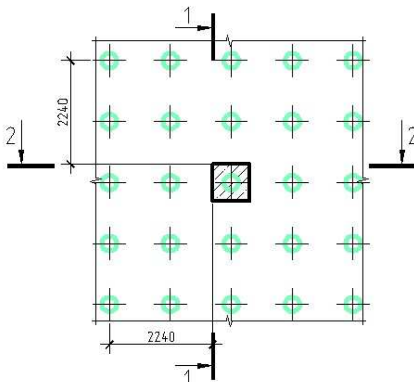
Рисунок 4.9 - Схема к расчету плиты на изгиб
