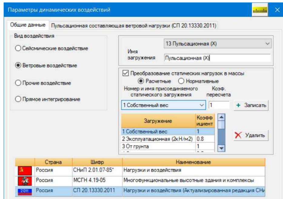
Рисунок 3.7 – Общие данные динамического воздействия
