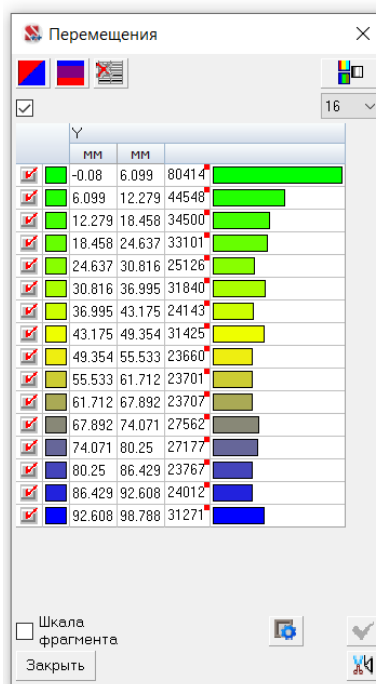
Рисунок 3.12 – Горизонтальные перемещения по оси Y
