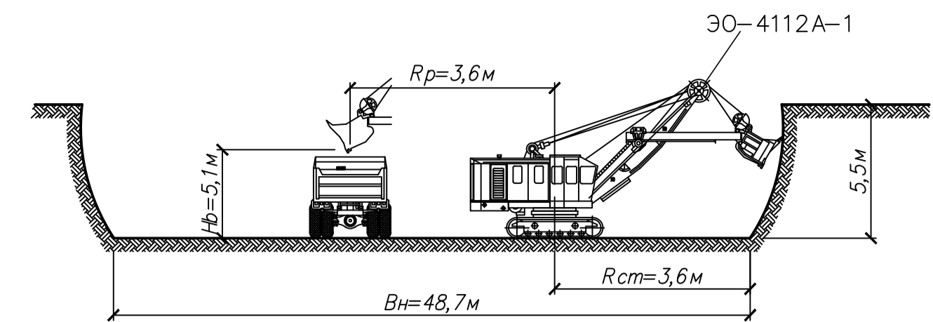
Схема разработки экскаваторами
