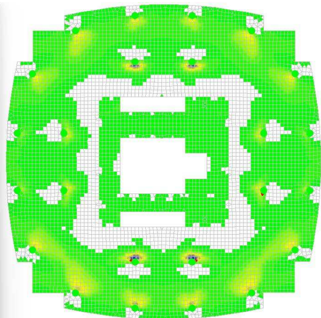
Рисунок 3.22 – Изополя армирования плиты интенсивность S_3 (нижня по Y)
