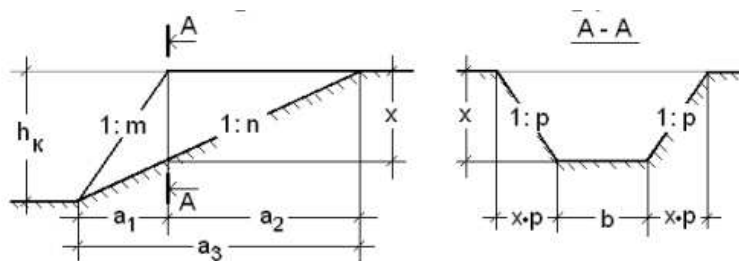
Рисунок 5.2 – Определение геометрического объема грунта съезда
