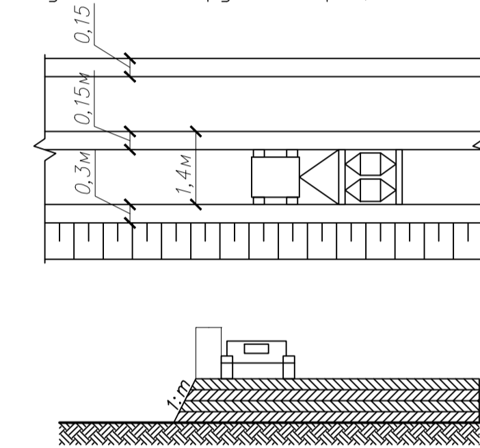
Схема уплотнения грунта вибрационным катком ДУ-32а
