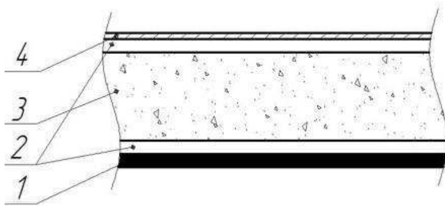
Рисунок 2 – Схема кровли
