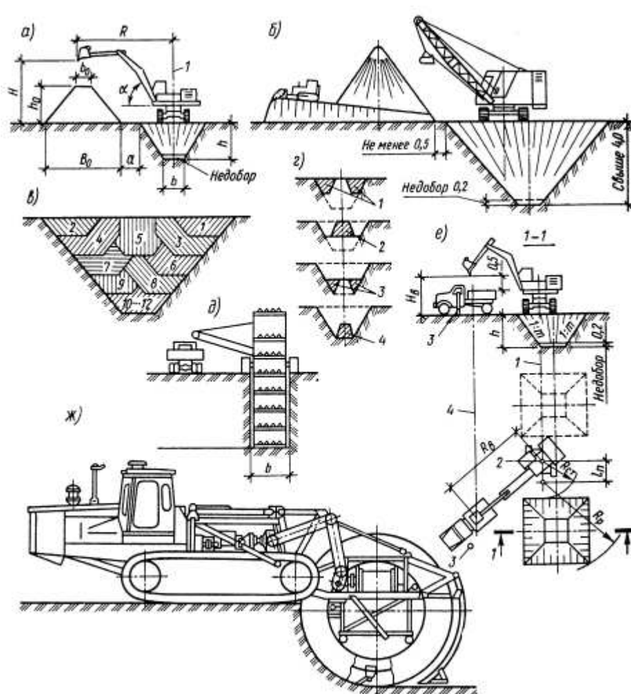
Рисунок 8.5 – Разработка траншей экскаватором
