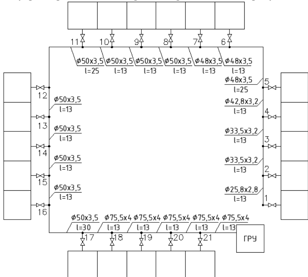
Рисунок 6.1 – Расчетная схема внутриквартирного газопровода
