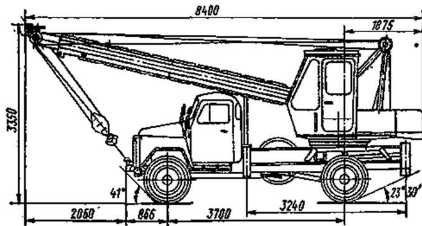
Рисунок 8.6 – Автокран марки КС-1562А
