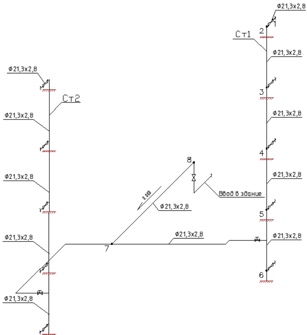
Рисунок 5.1– Расчетная схема внутридомового газопровода
