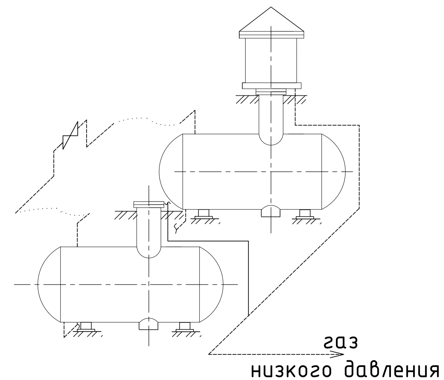
Схема обвязки резервуаров
