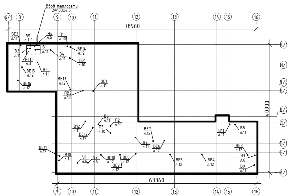
План-схема 1:400
