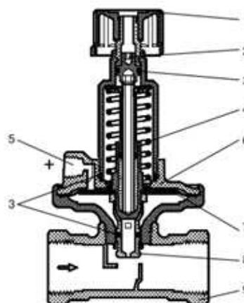
Устройство клапана ASV-PV D y = 15–40 мм
