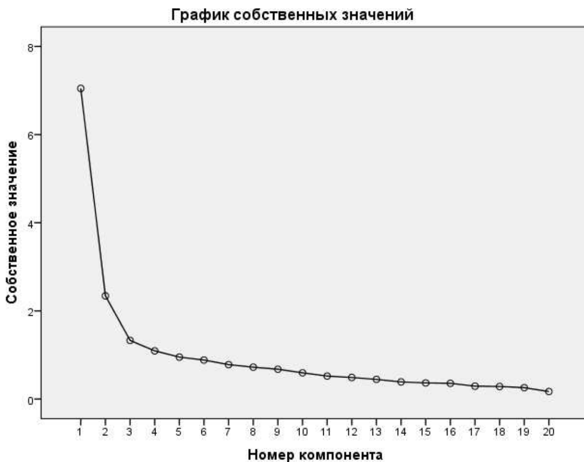
Рисунок 25 - График собственных значений
