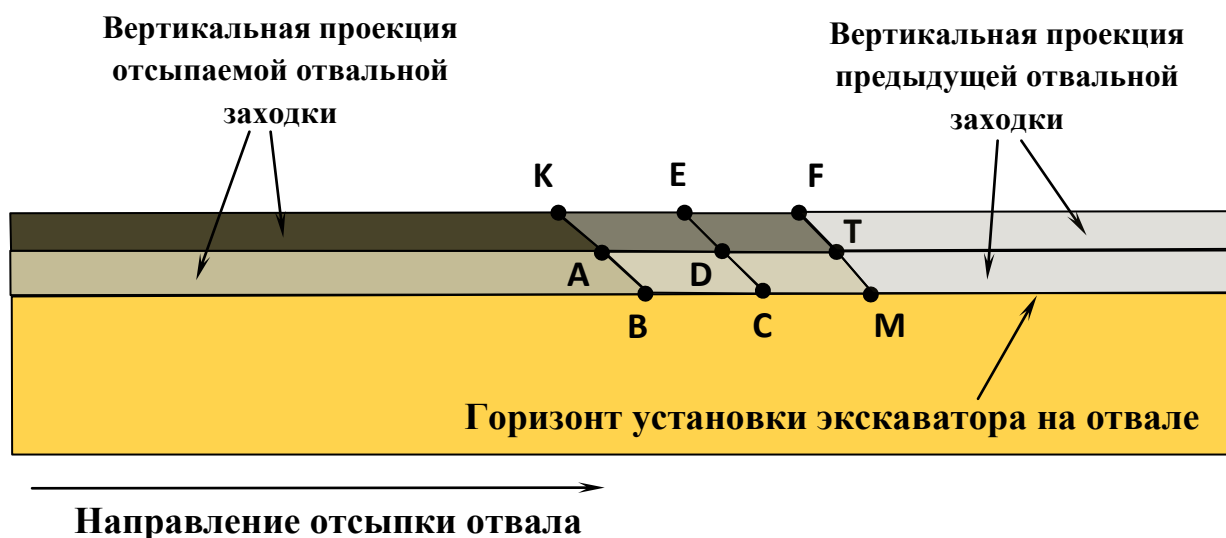
Рис. 5. Схема послойной отсыпки породного отвала по разработанной технологии при использовании железнодорожного транспорта
