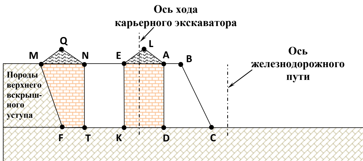
Рис. 4. Схема селективной отработки забоя верхнего вскрышного уступа карьерным экскаватором ЭКГ-10; ЭКГ-12,5
