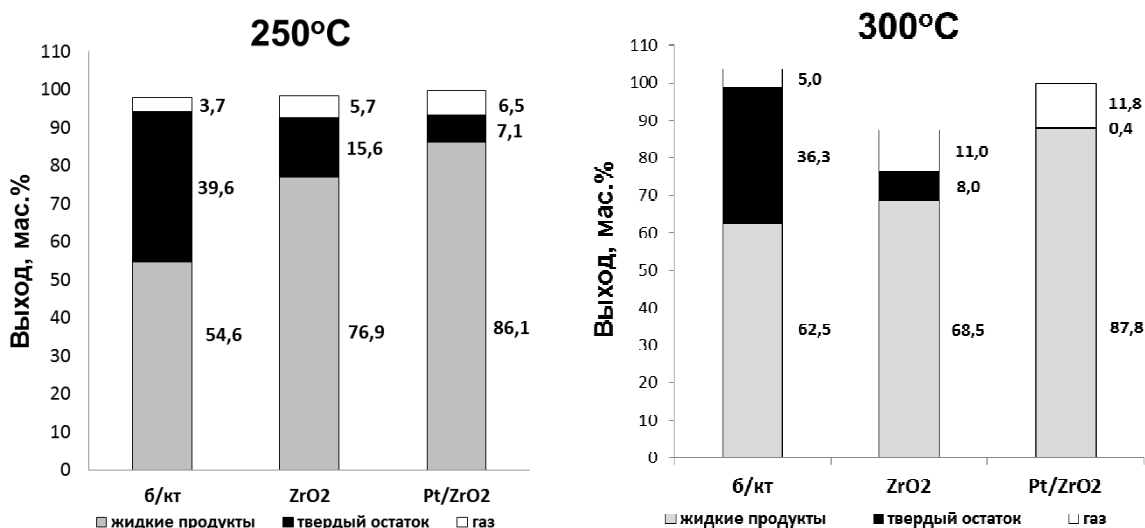
Рис. 2. Влияние катализаторов на выход продуктов гидрирования этанолигнина лиственницы в среде сверхкритического этанола при 250 и 300 °C (мас.%).
