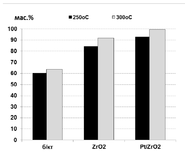
Рис. 1. Влияние катализаторов на конверсию этанолигнина лиственницы в процессе его гидрирования в среде сверхкритического этанола при 250 и 300°C (мас.%)
