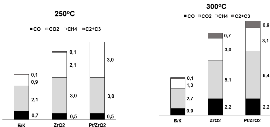
Рис. 3. Влияние катализаторов на выход газообразных продуктов гидрирования этаноллигнина лиственницы в среде сверхкритического этанола при 250 и 300 °С (мас.%).
