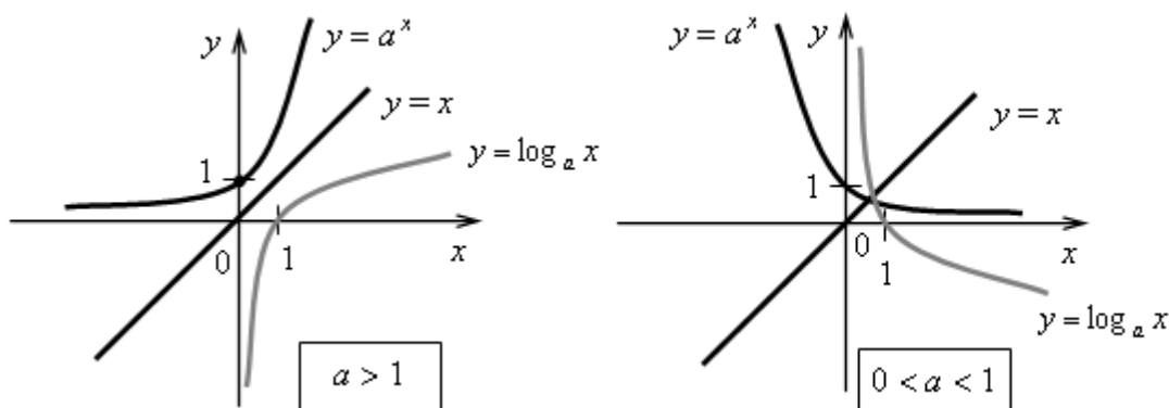
Рисунок 2 – графики логарифмической функции
