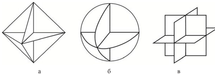
Рис. 4. Конструкции уголковых отражателей
