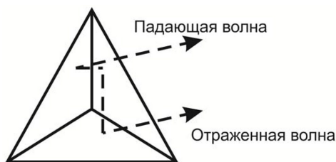
Рис. 5. Направления падающей и отраженной волн от углового отражателя
