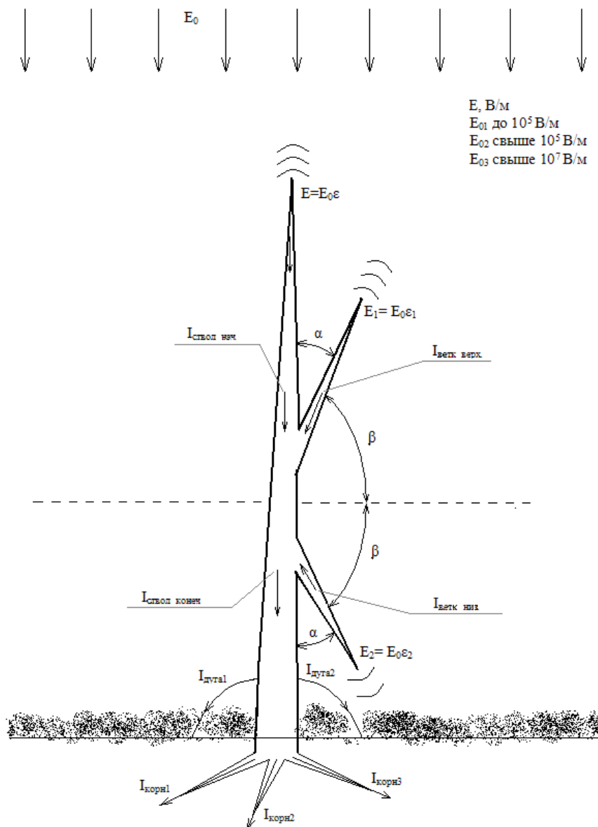
Рис. 1. Схема балансов электрических токов на участке «дерево-грунт» модели «грозовое облако-дерево»
