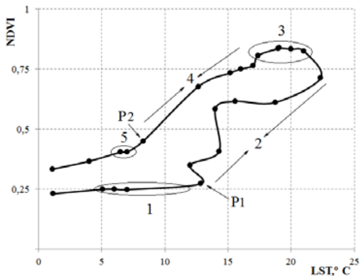
Рис. 3. Иллюстрация фазового портрета растительного объекта в пространстве (LST, NDVI). Цифры у кривой указывают фенологическую фазу: 1 – отсутствие вегетации, предвегетационный период; 2 – рост биомассы наземных органов (первый этап вегетационного периода); 3 – сезонный максимум биомассы; 4 – созревание семян, увядание листьев; 5 – послевегетационный период; P1, P2 – начало и окончание вегетации растительности
