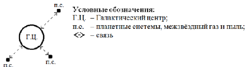
Рисунок 1.5. Условная модель «Галактики»
