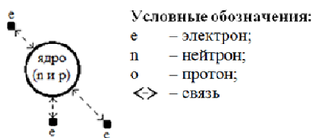
Рисунок 1.1. Условная модель строения атома химического элемента
