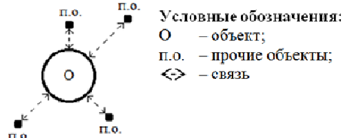
Рисунок 1.2. Условная модель «пространства» в определённый момент времени
