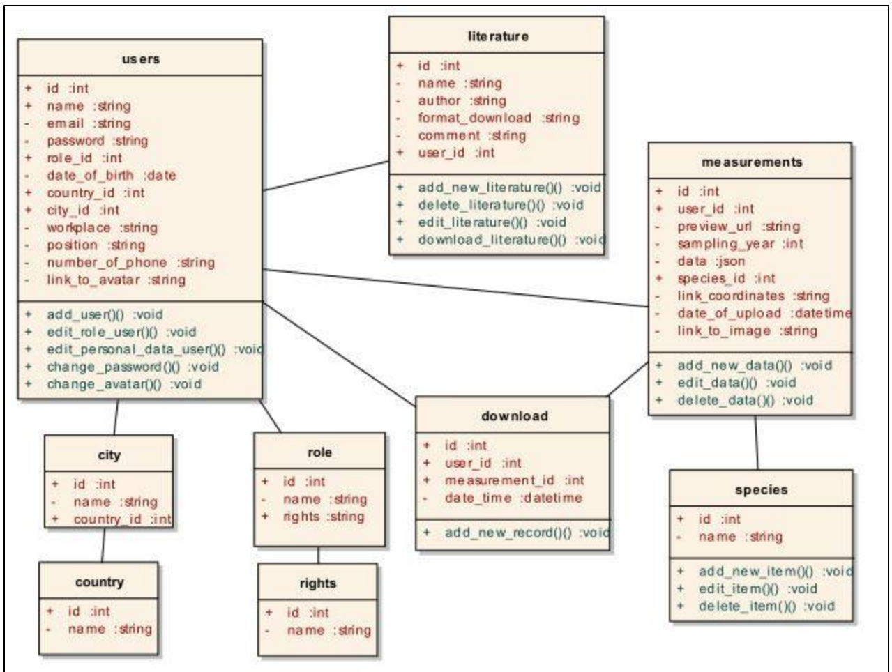
Рисунок 10 — Диаграмма классов
