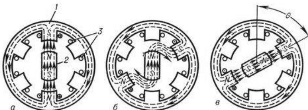
Рисунок 5—Основные стадии работы шагового двигателя
