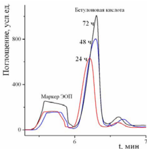
Рис. 2. Электрофореграммы бетулоновой кислоты, полученные через 24-72 ч перемешивания в 40 мМ растворе ГП-γ-ЦД
