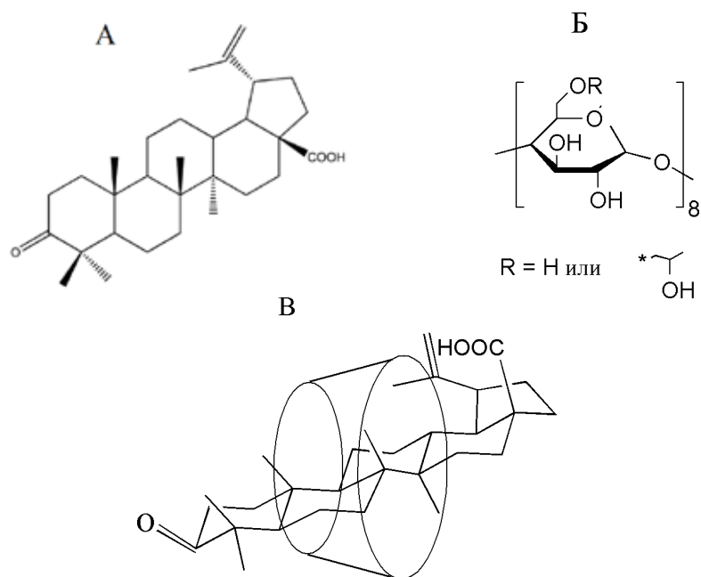
Рис. 1. Структурные формулы бетулоновой кислоты (А), ГП-γ-ЦД (Б) и образованного ими комплекса (В)
