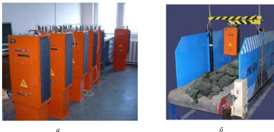
Рис. 2. РКС-КМ : а – заводские испытания РКС; б – сбор на ленточном конвейере
