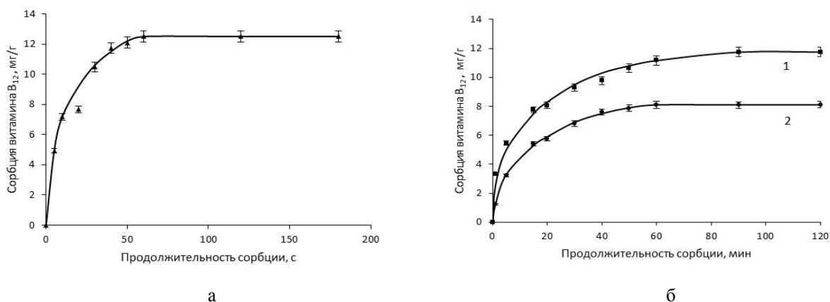
Рис. 3. Кинетика сорбции витамина \text{B}_{12} на углеродных сорбентах из коры осины и активированном угле УА–Н: а – сорбент из коры осины СКО–1; б – сорбент из коры осины СКО–3 (1) и активированный уголь УА–Н (2)
