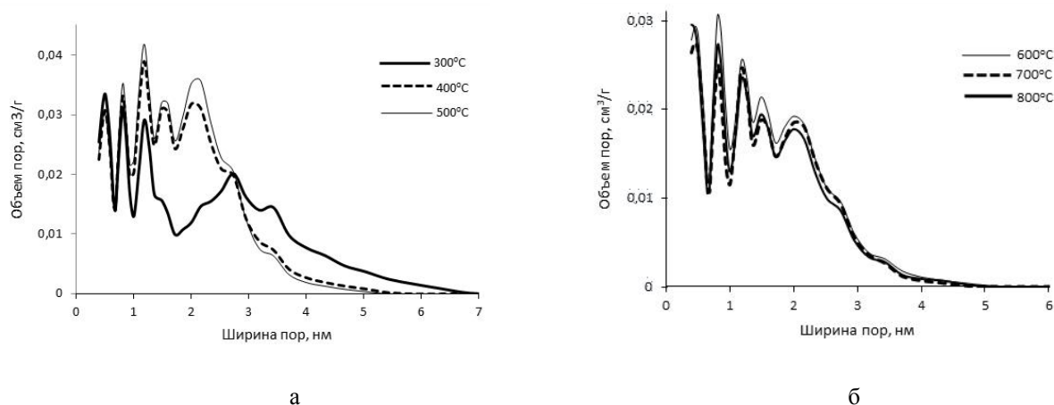
Рис. 1 Распределение пор по размерам в углеродных сорбентах из коры осины в зависимости от температуры получения исходных карбонизатов: а – температуры 300, 400 и 500 °С; б – температуры 600, 700 и 800 °С
