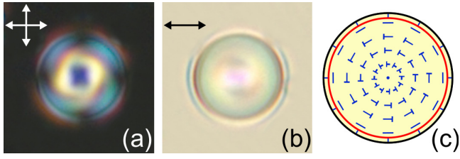
Рис. 1. Фотографии капли с тороидальной структурой холестерика, когда ось симметрии капли перпендикулярна плоскости образца, сделанные в геометрии скрещенных поляризаторов (а) и с выключенным анализатором (б). Схематическое представление линий директора в центральном сечении капли (с). Направления поляризаторов здесь и далее обозначены двойными стрелками, красная линия обозначает кольцевой поверхностный дефект. Диаметр капли 11 мкм, собственный шаг спирали холестерика p_0 = 5.5 мкм.
