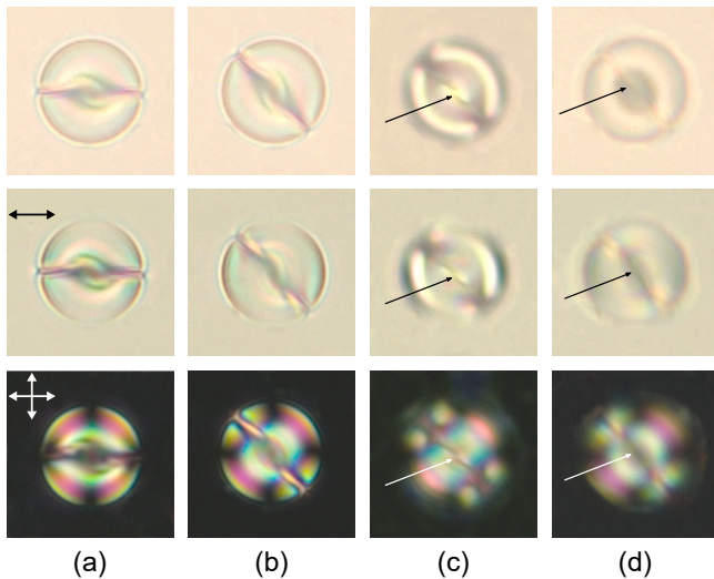
Рис. 2. Фотографии капли с тороидальной структурой холестерика, когда ось симметрии капли лежит в плоскости композитной пленки. Ось симметрии капли перпендикулярна поляризатору (а) и ориентирована к нему под углом 45^\circ в случае, когда микроскоп сфокусирован на центр капли (б), на участок кольцевого дефекта, расположенного выше (с) и ниже (д) центра капли. Фотографии сделаны в неполяризованном свете (верхний ряд), в схеме с выключенным анализатором (средний ряд) и в скрещенных поляризаторах (нижний ряд). Одинарными стрелками показано положение кольцевого дефекта. Диаметр капли 11 мкм.
