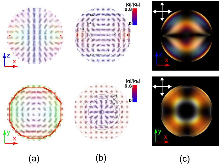
Рис. 3. (a) Рассчитанная конфигурация директора в капле с тороидальной структурой холестерика, имеющей кольцевой поверхностный дефект в центральном сечении. Распределение поля директора раскрашено в соответствии с направлением по отношению к осям: красный – Ox , зеленый – Oy , синий – Oz , кольцевой дефект обозначен жирной красной линией. (b) Поле волнового вектора \mathbf{q} холестерической спирали, раскрашенное в соответствии с относительной длиной |\mathbf{q}|/|\mathbf{q}_0| , контурными линиями обозначены границы областей с соотношением |\mathbf{q}|/|\mathbf{q}_0| < 1/6 , |\mathbf{q}|/|\mathbf{q}_0| < 2/6 и |\mathbf{q}|/|\mathbf{q}_0| < 4/6 . (c) Смоделированные оптические текстуры в геометрии скрещенных поляризаторов. Диаметр капли 11.8 мкм.
