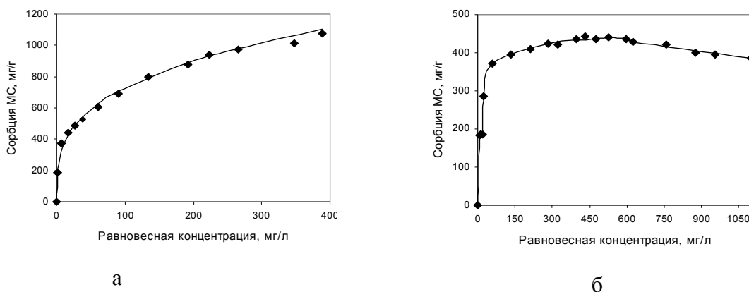
Рис. 5. Изотермы сорбции метиленового синего (МС) для углеродных сорбентов из лигнина ЭЛ – 5 (а) и ЭЛ – 8 (б): точки – экспериментальные значения; линия на рис. 5-а – результаты расчета по уравнению Фрейндлиха.
