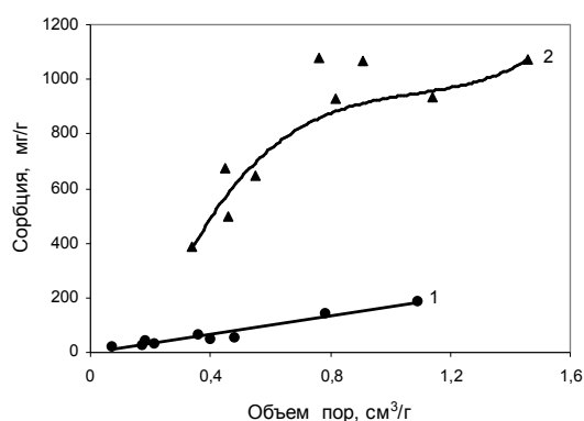
Рис. 3. Зависимость сорбции витамина В 12 (1) и метиленового синего (2) от объема пор сорбентов из лигнина: 1 – от объема пор шириной 1,69 – 3,61 нм; 2 – от объема пор шириной 1,06 – 3,61 нм.
