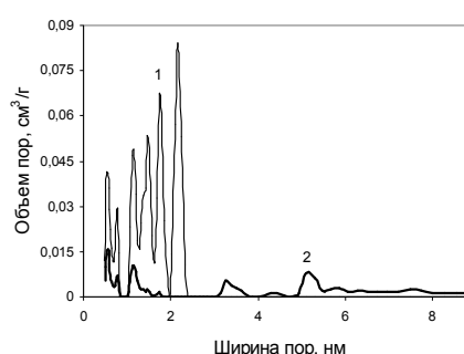
Рис. 2. Распределение пор по размерам для сорбента из лигнина ЭЛ – 6 (1) и активного угля УА-Н (2)
