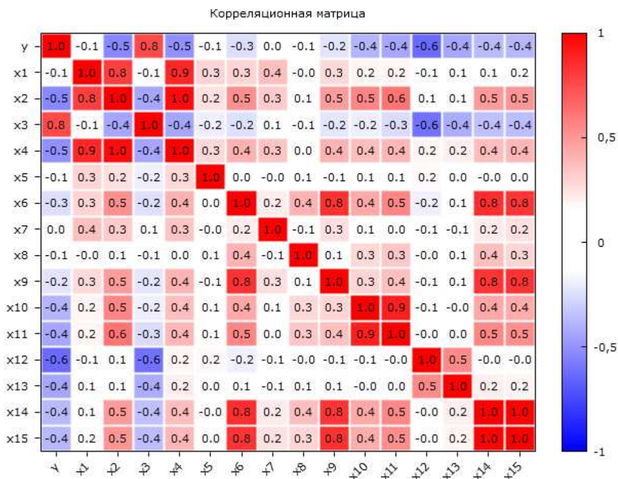
Рисунок 8 – Корреляционная матрица 15 регрессоров
