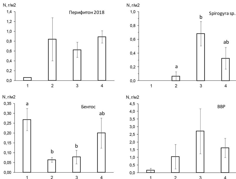
Рис. 9. Средние значения содержания общего азота ( \text{г}/\text{м}^2 ) в биомассе фитоперифитона (2018 г.), зообентоса, Spirogyra sp. (метафитон) и высших водных растений (ВВР) (2018-2019 гг.) в Абаканской протоке р. Енисей. Средние, отмеченные одинаковыми буквами, достоверно не отличаются по критерию Краскела-Уоллиса. При недостоверном критерии буквенные обозначения отсутствуют
